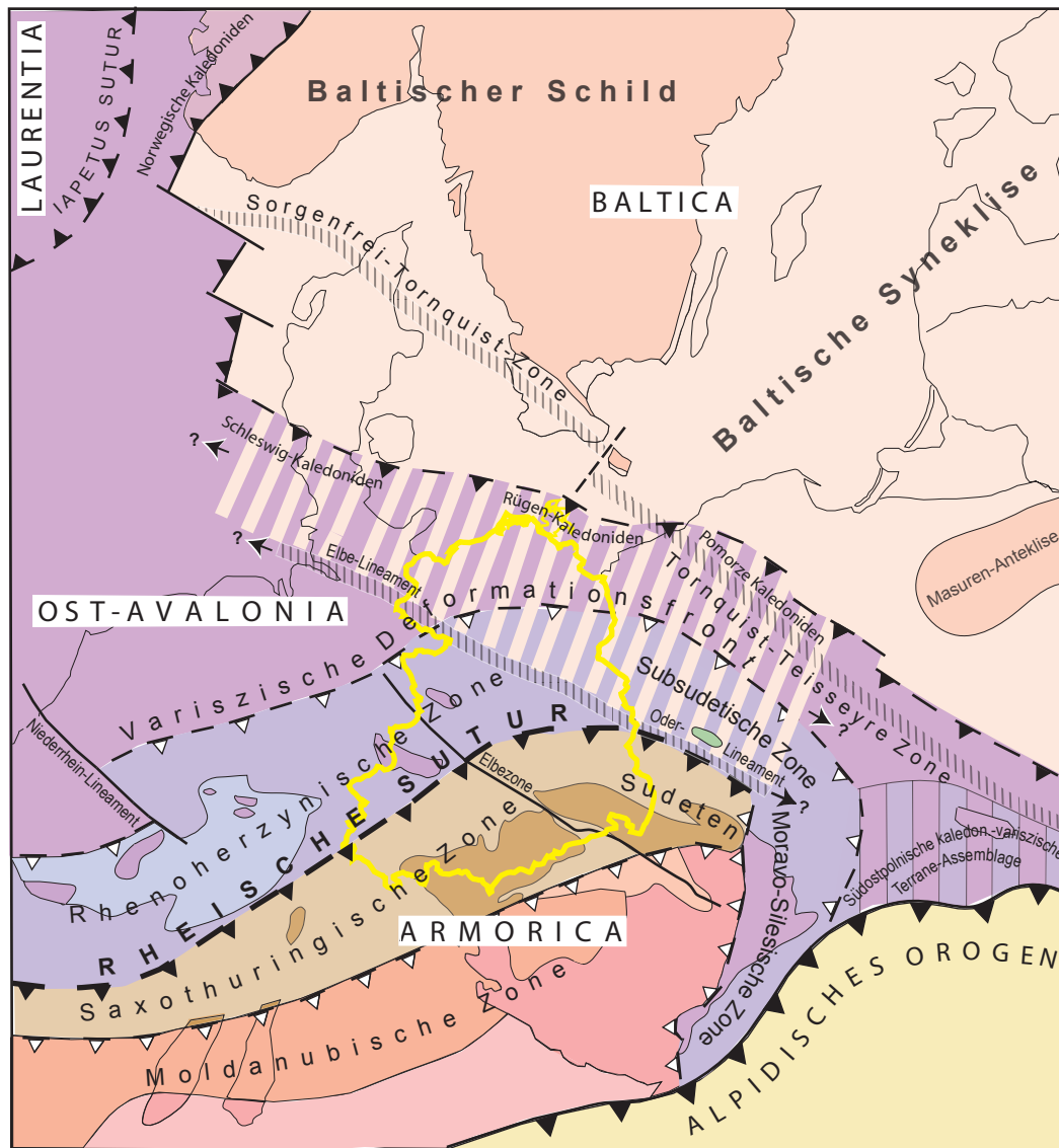
Abb. 1.1 Die Position Ostdeutschlands (gelbe Grenze) im tektonischen Bauplan Mitteleuropas (nach T. McCANN & M. KRAWCYK 2001; J.A. WINCHESTER et al. 2002; P.A. ZIEGLER & P. DEZES 2005; R. WALTER 2007; C.M. KRAWCYK et al. 2008; D. FRANKE & W. STACKEBRANDT 2015)
