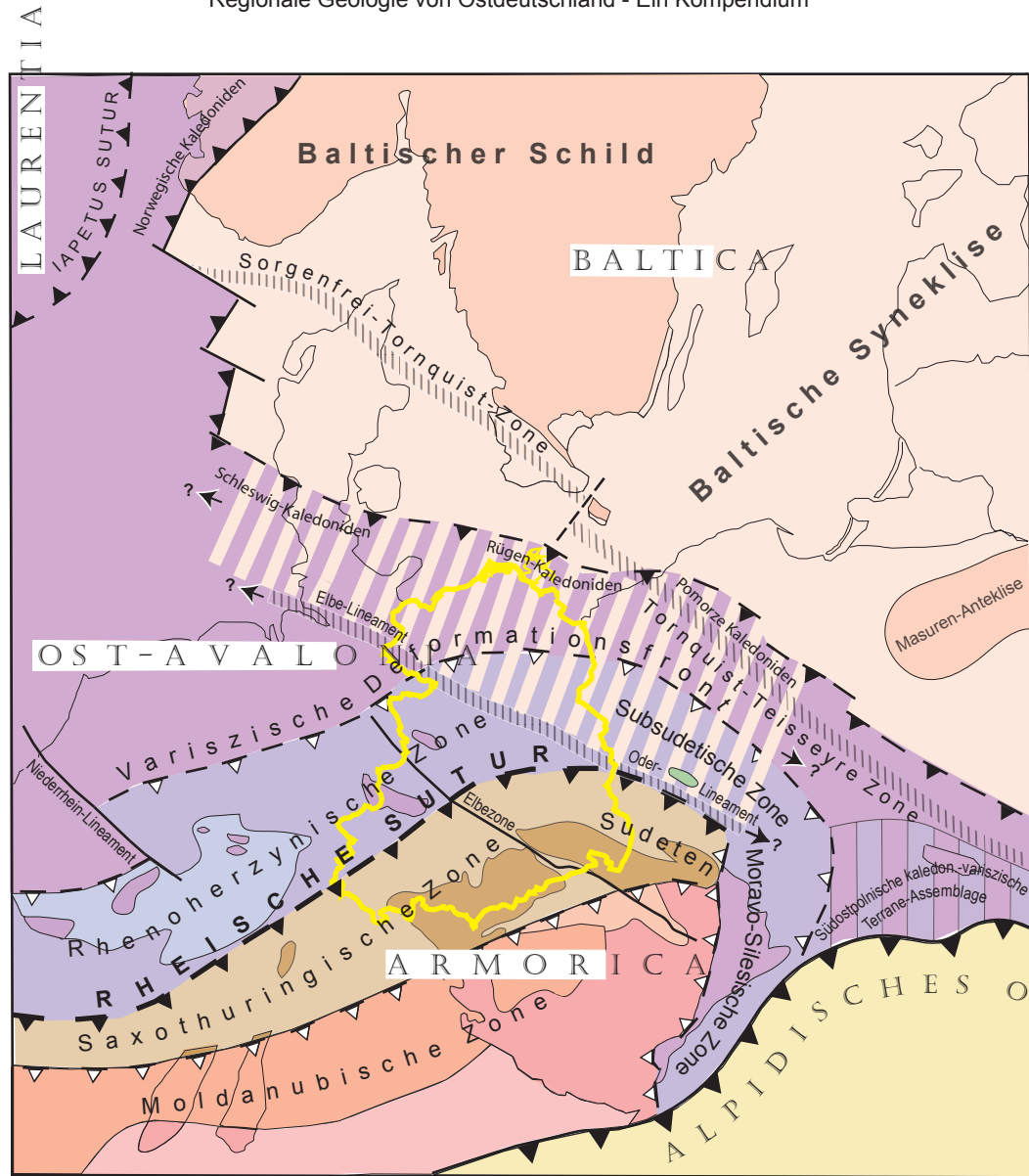
Abb. 1.1 Die Position Ostdeutschlands (gelbe Grenze) im tektonischen Bauplan Mitteleuropas (nach T. McCANN & M. KRAWCYK 2001; J.A. WINCHESTER et al. 2002; P.A. ZIEGLER & P. DEZES 2005; R. WALTER 2007; C.M. KRAWCYK et al. 2008; D. FRANKE & W. STACKEBRANDT 2015)
