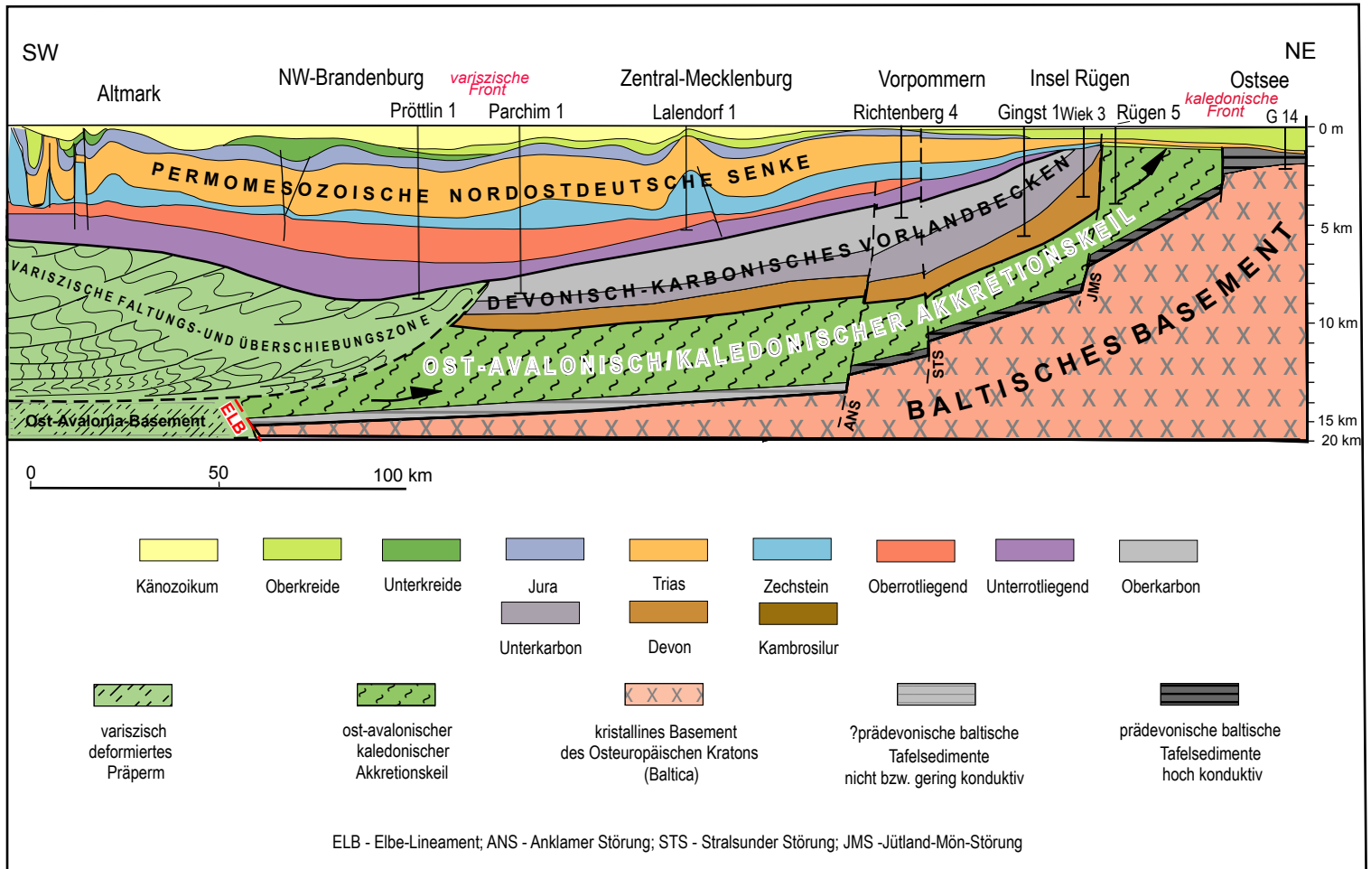
Abb. 1.2 Geologisch-tektonischer Schnitt von der variszischen Außenzone über die Rügen-Kaledoniden bis zum Südwestrand Balticas
