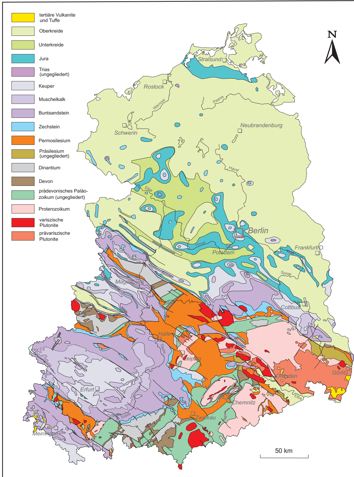
Abb. 2 Geologische Übersichtskarte von Ostdeutschland ohne känozoische Sedimente (nach G. RÖLLIG et al. 1990; D. LEONHARDT 1995; G. MARTIKLOS et al. 2001; G. SEIDEL et al. 2002)
