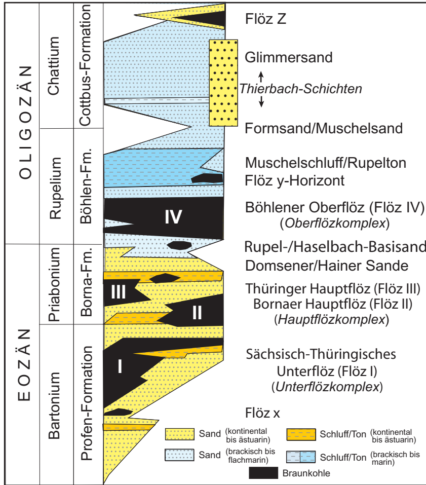
Abb. 23.10 Profilentwicklung im Bereich des Leipzig-Borna-Altendburger Tertiärgebietes ("Weißelster-Becken") (nach J. RASCHER et al. 2005; G. STANDKE 2008b; W. KRUTZSCH 2011)
