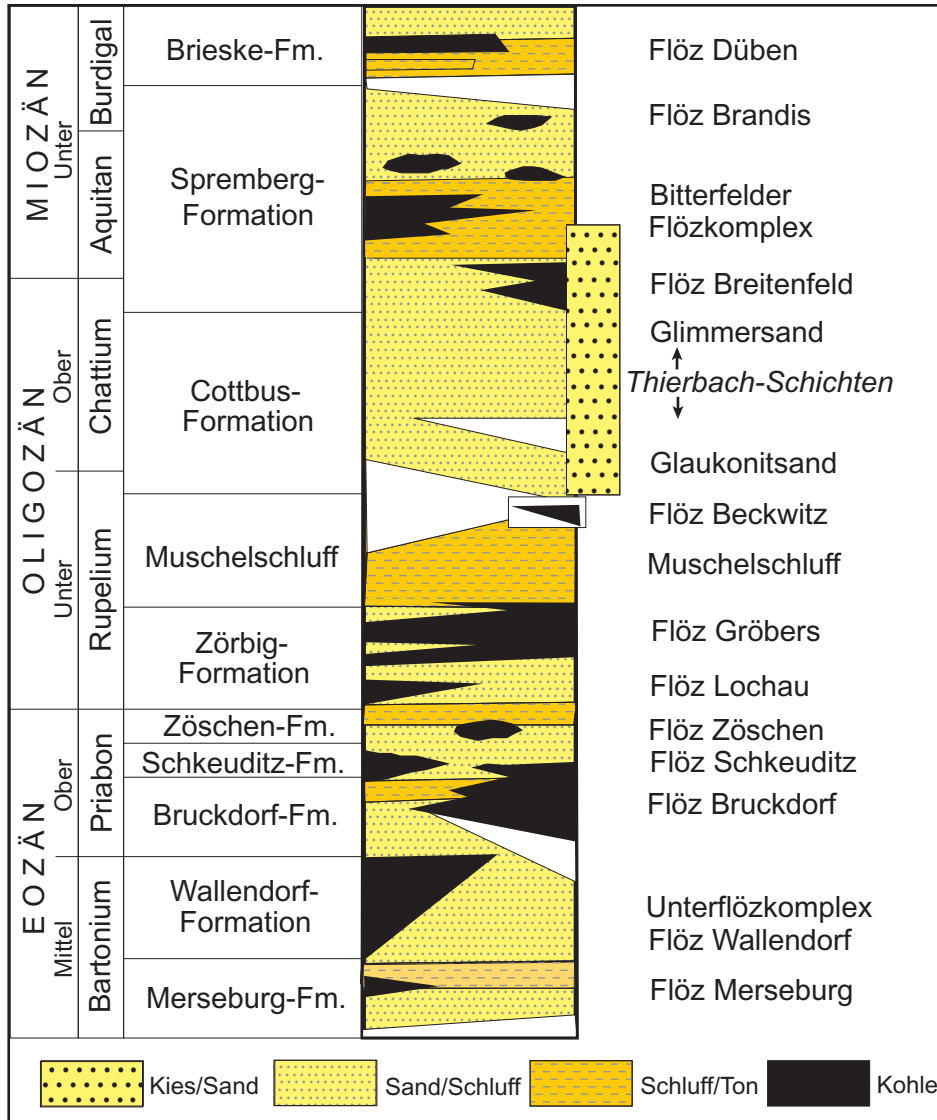
Abb. 23.11 Profilentwicklung des Tertiär im Bereich des Halle-Merseburger Tertiärgebietes (nach J. RASCHER et al. 2005)
