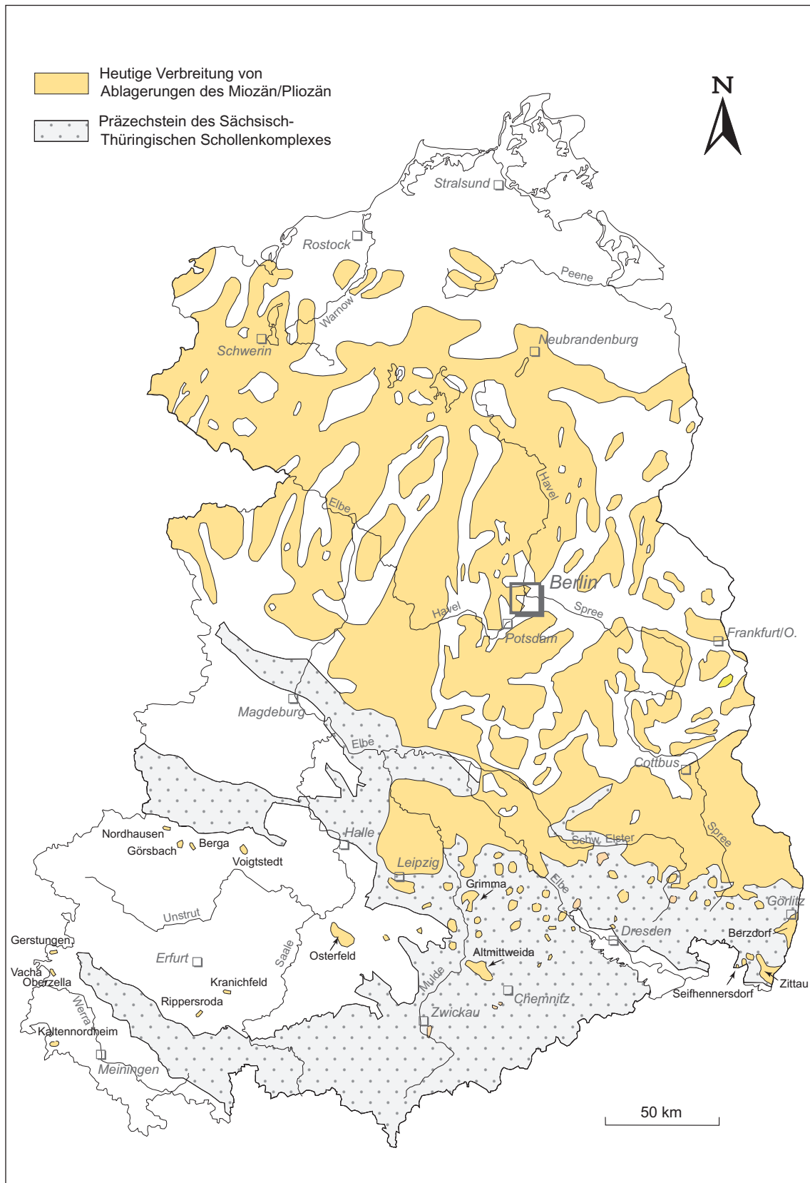
Abb. 23.4 Heutige Verbreitung von Ablagerungen des Miozän/Pliozän in Ostdeutschland (generalisierte Darstellung nach W. ALEXOWSKY 1994; J. HAUPT 1996; H. JORTZIG 2002; G. MARTIKLOS 2002a)
