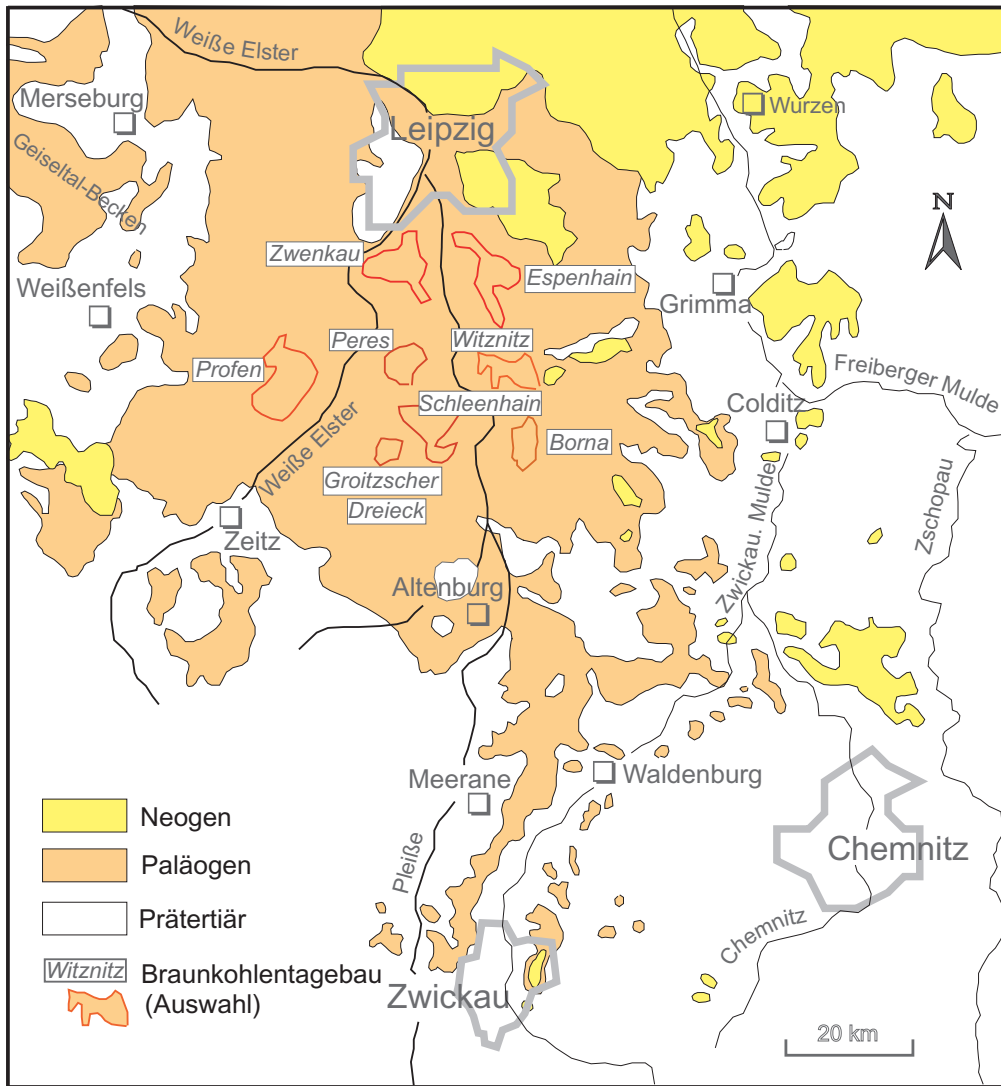
Abb. 23.5 Geologie des Leipzig-Borna-Altenburger Tertiärgebietes ("Weißelster-Becken") (nach W. ALEXOWSKY 1994; G. STANDKE & P. SUHR 1998)
