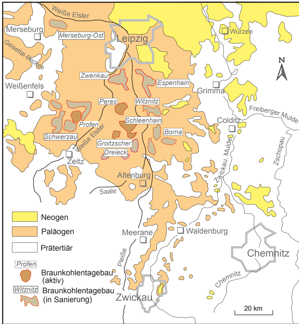
Abb. 23.5 Geologie des Leipzig-Borna-Altenburger Tertiärgebietes ("Weißelster-Becken") (nach W. ALEXOWSKY 1994; G. STANDKE & P. SUHR 1998; J. RASCHER et al. 2013)
