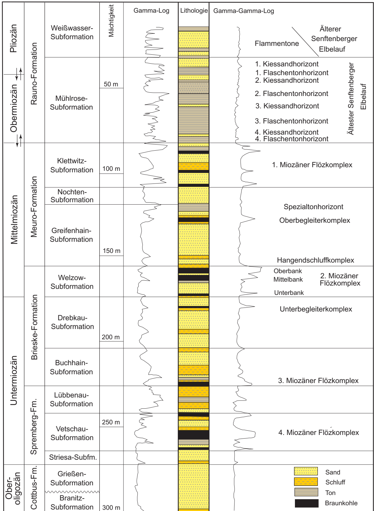
Abb. 23.7 Lithostratigraphisches Richtprofil für das Tertiär des Niederlausitzer Tertiärgebiets
