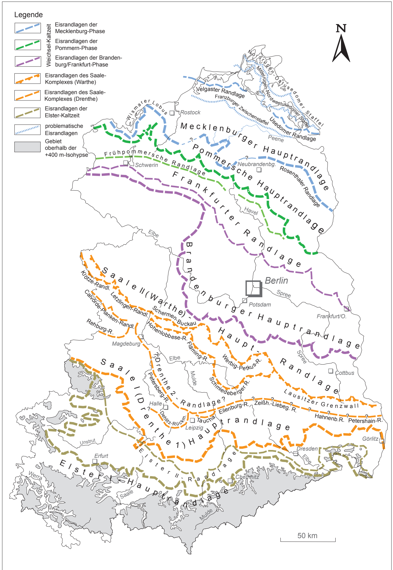
Abb. 24.1 Position bedeutender Eisrandlagen des Pleistozän in Ostdeutschland (nach A.G. CEPEK 1968; J. MARCINEK & B. NITZ 1973; W. KNOTH 1995; L. EISSMANN 1997a; L. LIPPSTREU 2002b; F. BREMER 2004; T. LITT et al. 2007; K. SCHUBERTH 2008; L. WOLF & W. ALEXOWSKY 2008; L. LIPPSTREU et al. 2015)
