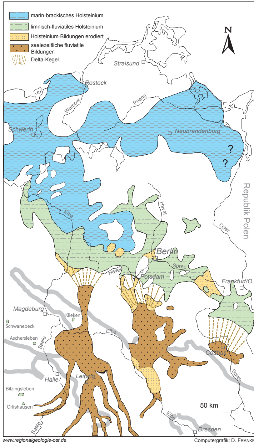
Abb. 24.2 Heutige Verbreitung von Ablagerungen der Holstein-Warmzeit sowie saalezeitlicher Terrassenbildungen in Ostdeutschland
