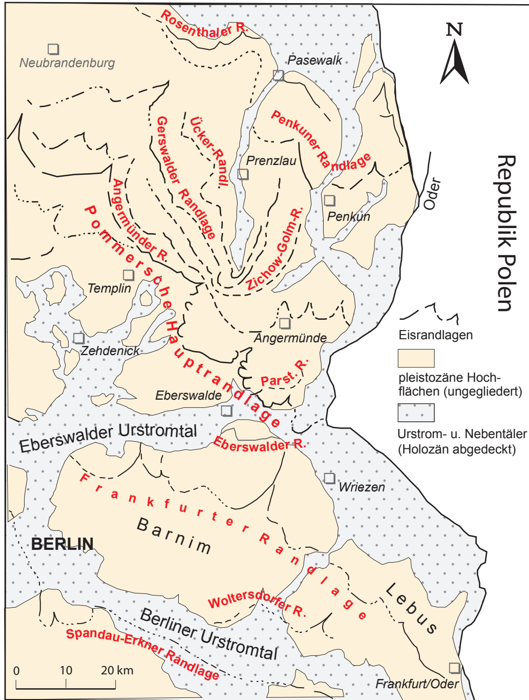
Abb. 24.3 Eisrandlagen der Weichsel-Kaltzeit in Nordostbrandenburg (nach A.G. CEPEK 1994, L. LIPPSTREU et al. 2015)
