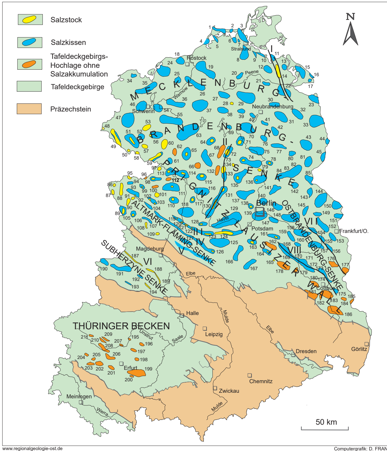
Abb. 25.1 Salinarstrukturen und Hochlagen ohne Salzakkumulation im Tafeldeckgebirge Ostdeutschlands (nach G. LANGE et. al. 1990; D. HÄNIG et al. 1996, 1997; N. RÜHBERG 1997; H. BEER 2000; G. BEUTLER 2001; P. KRULL 2004a; L. STOTTMEISTER et al. 2008)
