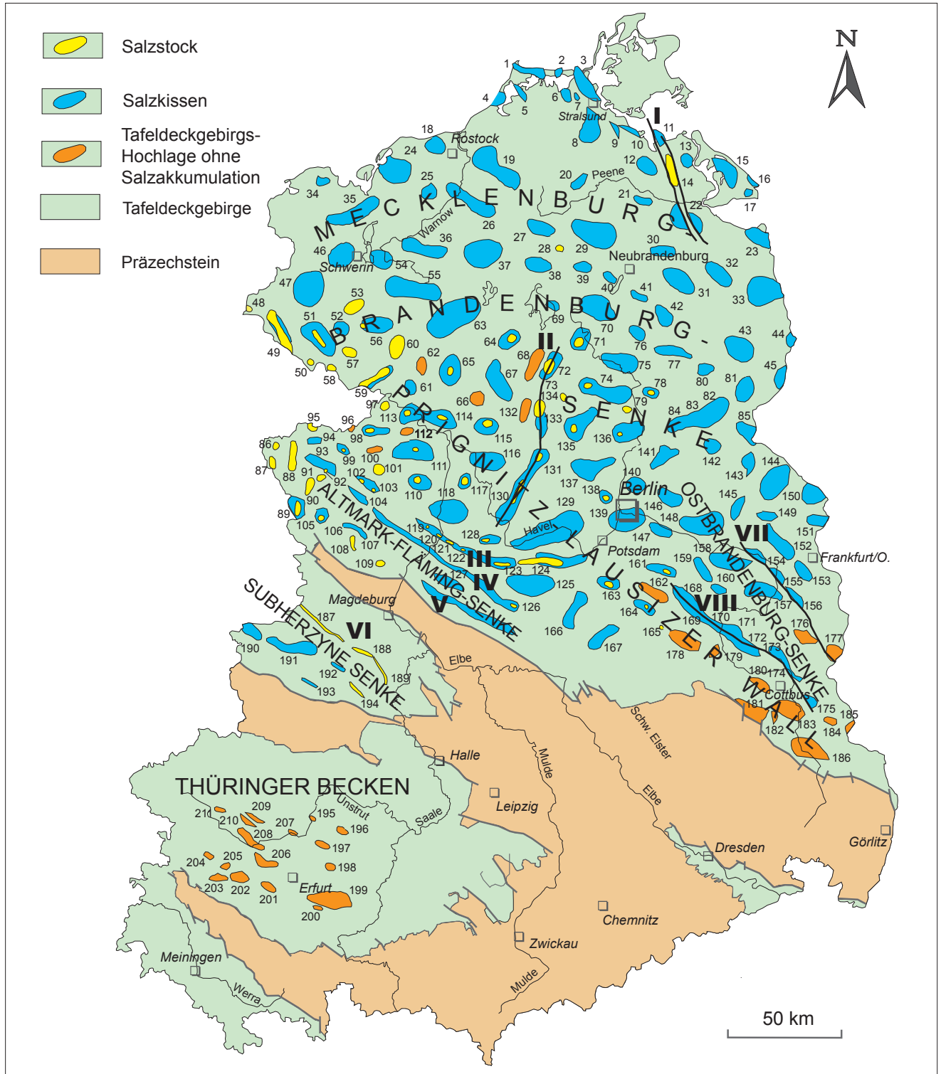
Abb. 25.1 Salinarstrukturen und Hochlagen ohne Salzakkumulation im Tafeldeckgebirge Ostdeutschlands
