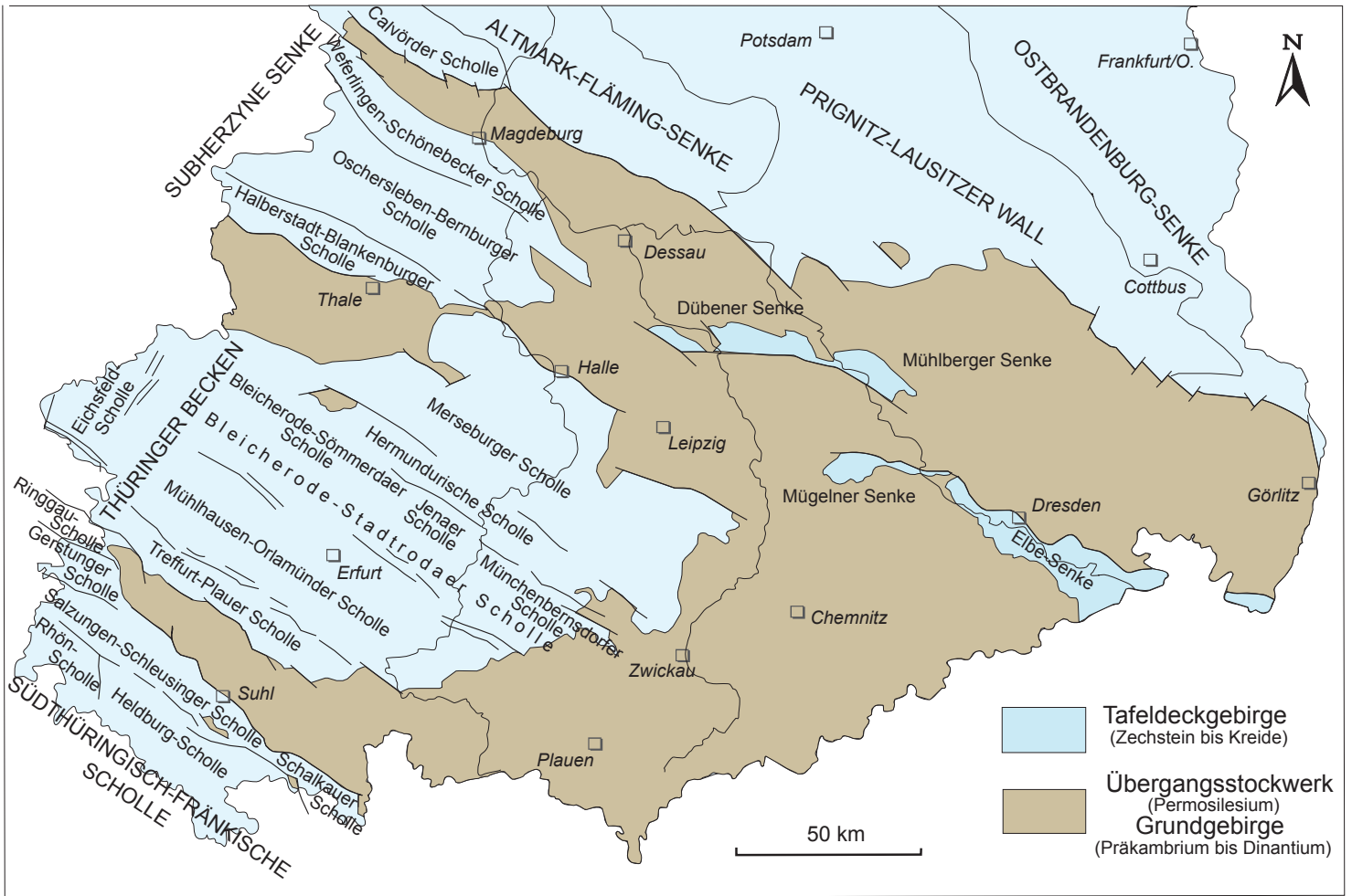
Abb. 25.10 Senken und Schollen des Tafeldeckgebirge im Südteil Ostdeutschlands (nach Geologie-Standard TGL 34331/01 1983; publiziert in G. KATZUNG & G. EHMKE/Hrsg. 1993; G. SEIDEL 2003, 2004)
