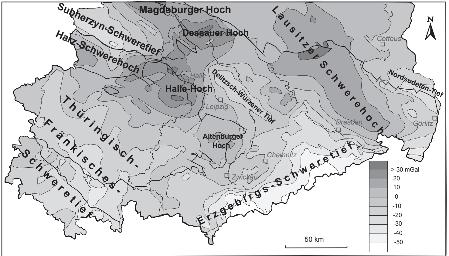
Abb. 25.11 Isanomalien der Bouguerschwere im Südteil Ostdeutschlands (nach W. CONRAD et al. 1994; D. HÄNIG et al 1996; W. CONRAD 1996; W. LANGE & I. RAPPSILBER 2008) Detaildarstellung der Lokalfeldanomalien vgl. Abb. 3.4
