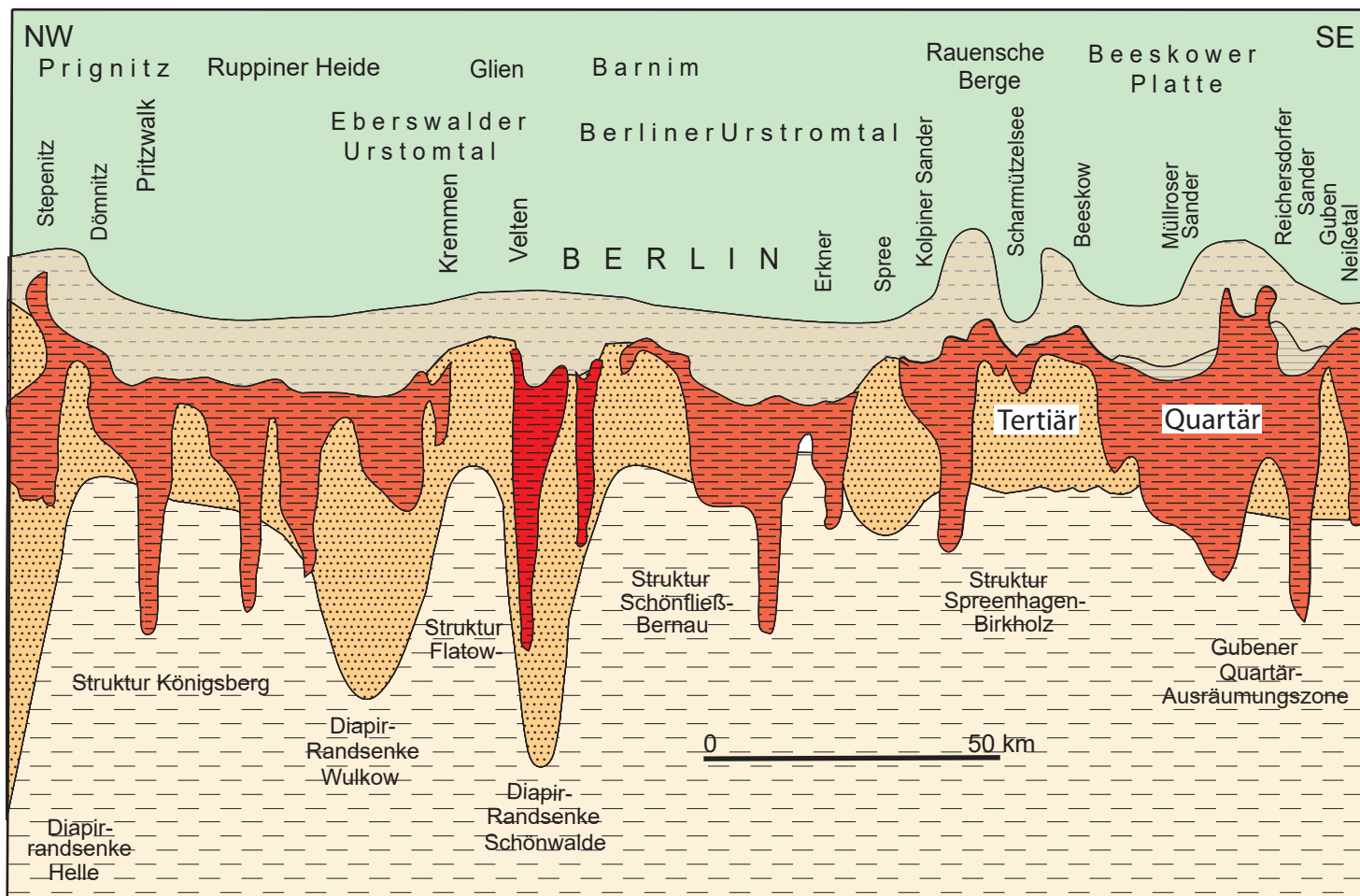
Abb. 25.12.3 Schnitt durch das jüngere Känozoikum Brandenburgs zwischen Prignitz und Neißetal (stark überhöht)
