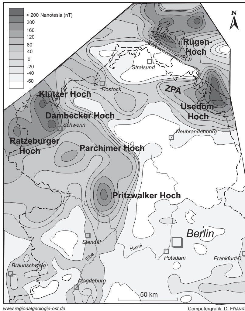
Abb. 25.17 Isanomalien des Magnetfeldes \Delta T im Bereich der Nordostdeutschen Senke in 700 m Höhe
