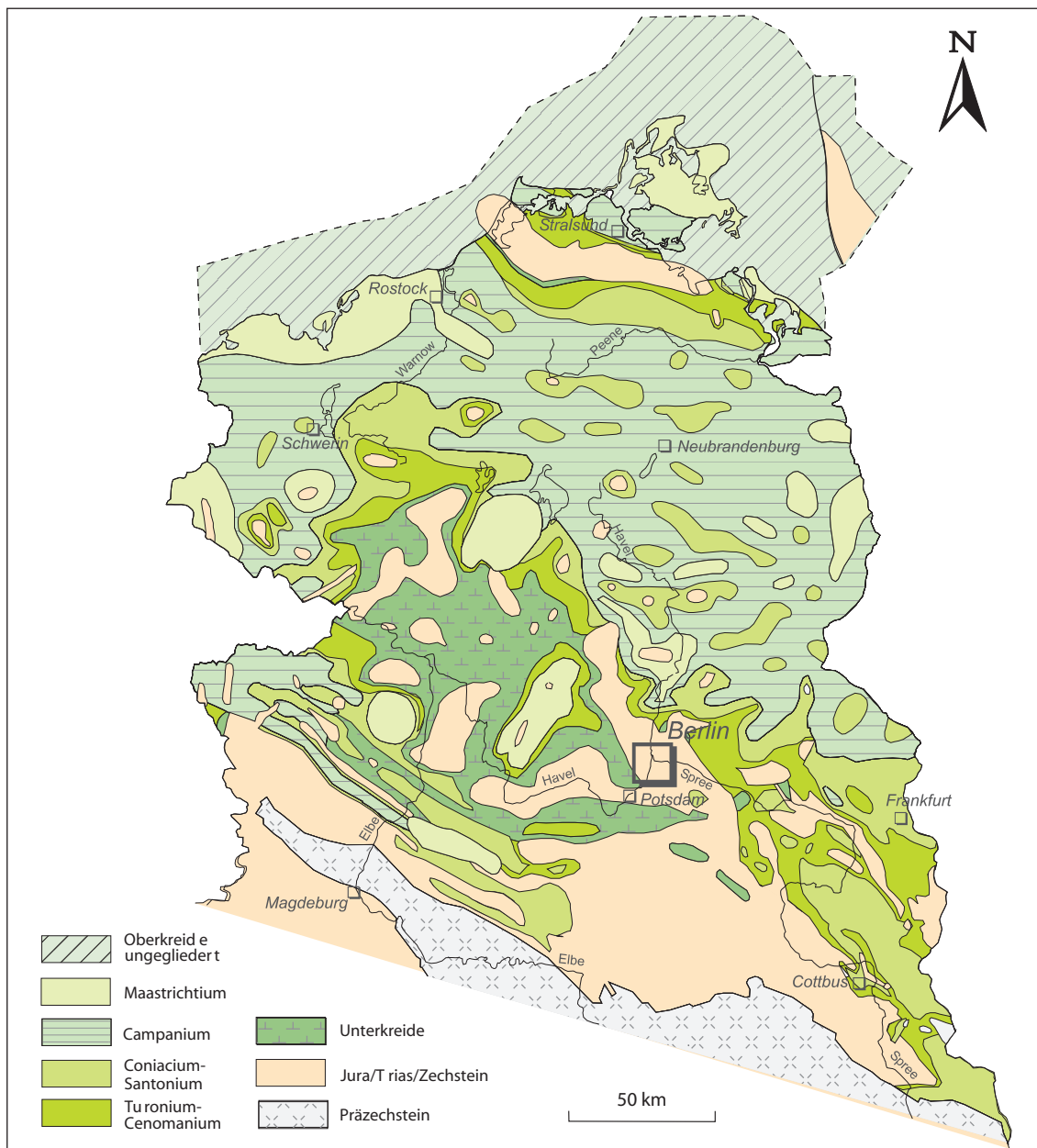
Abb. 25.1 Verbreitung von Ablagerungen der Oberkreide an der Oberfläche des Präkämzoikum im Bereich der Nordostdeutschen Senke
