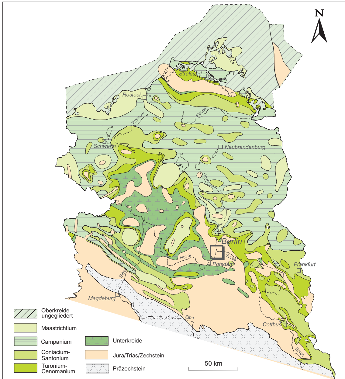
Abb. 25.2 Verbreitung von Ablagerungen der Oberkreide an der Oberfläche des Präkämzoikum im Bereich der Nordostdeutschen Senke
