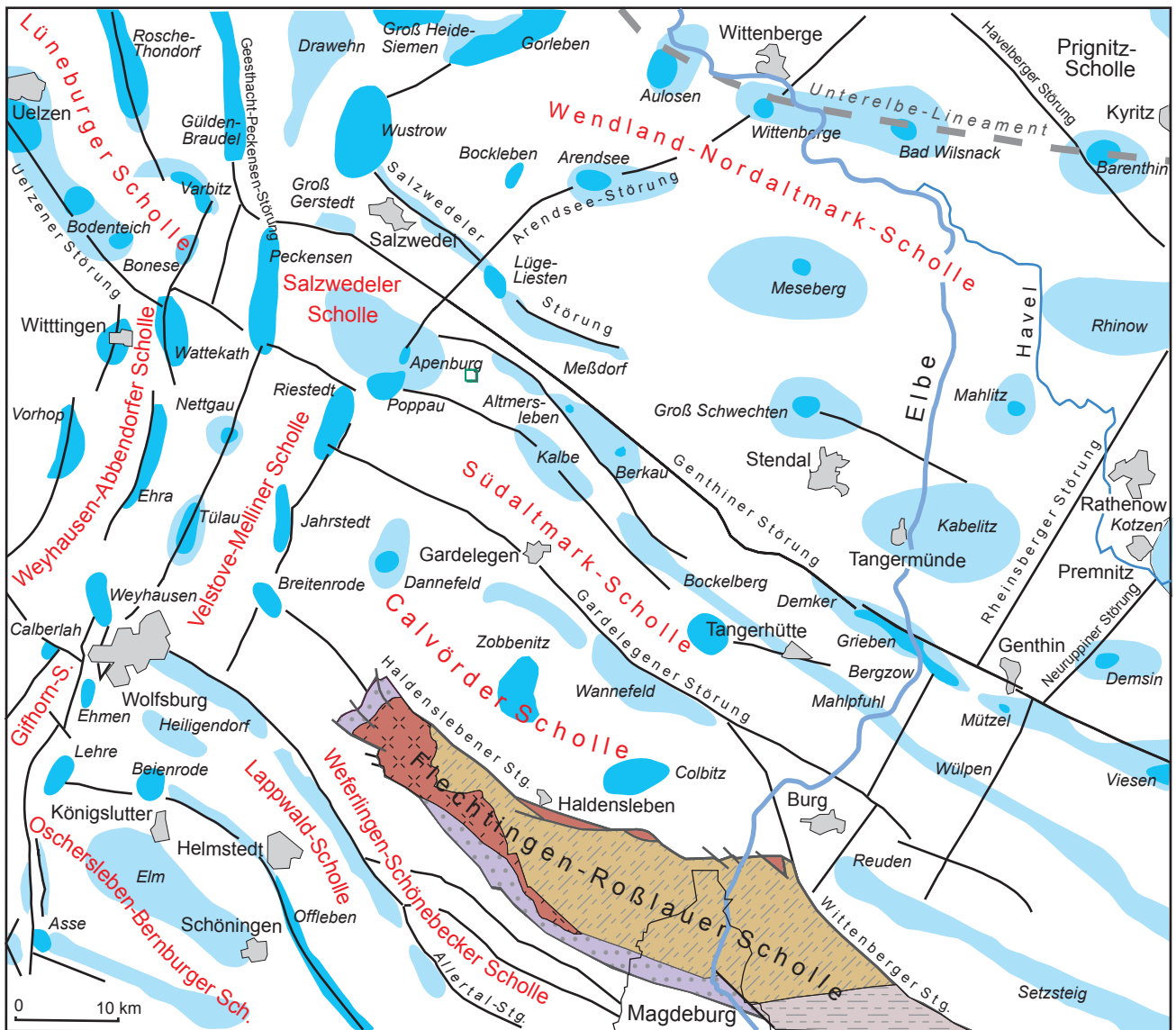
Abb. 25.20 Regionale Gliederung der Altmark-Fläming-Scholle und angrenzender Bereiche mit Darstellung der wichtigsten Salinarstrukturen (Salzstöcke dunkelblau, Salzkissen hellblau)
