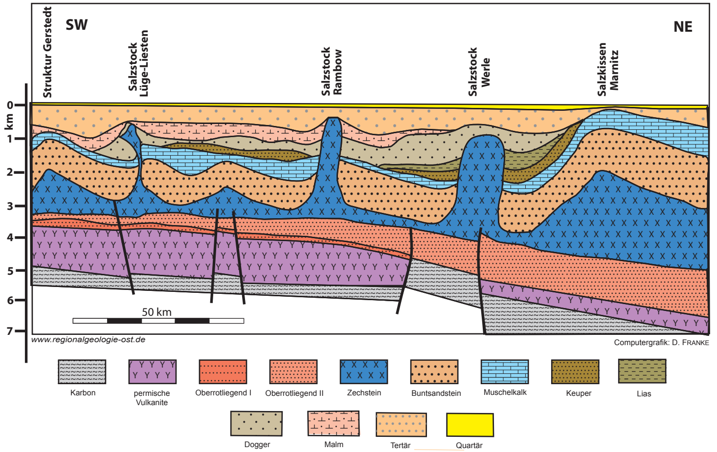
Abb. 25.22.1 Zechstein-Salzstrukturen am Nordwestrand von Brandenburg (nach M. WOLFGGRAMM 2005)
