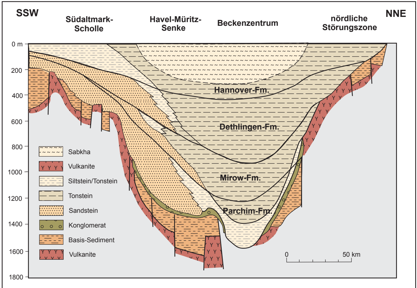
Abb. 25.23 SSW-NNE-Schnitt durch das nordostdeutsche Rotliegendebcken
