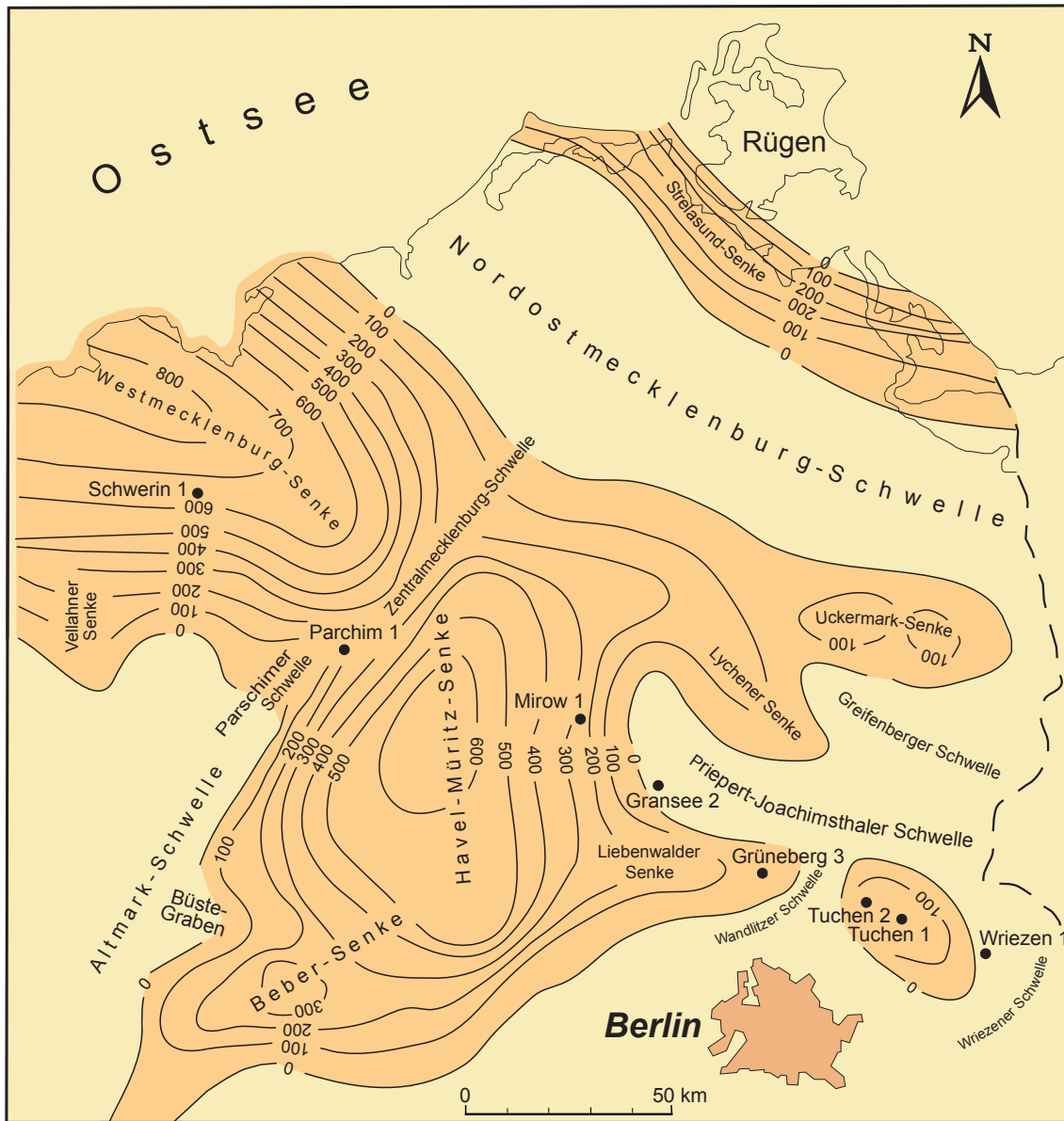
Abb. 25.24 Verbreitung und Mächtigkeit der Parchim-Formation des Rotliegenden im Bereich der Nordostdeutschen Senke (nach W. LINDERT et al. 1990)
