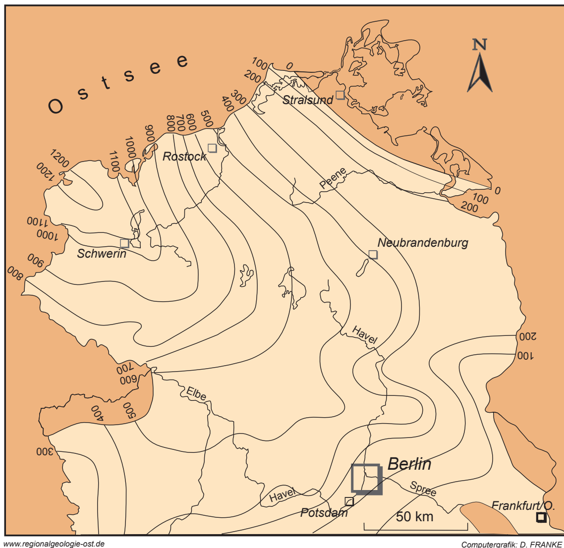
Abb. 25.26 Verbreitung und Mächtigkeit von Schichtenfolgen der Elbe-Subgruppe im Bereich der Nordostdeutschen Senke
