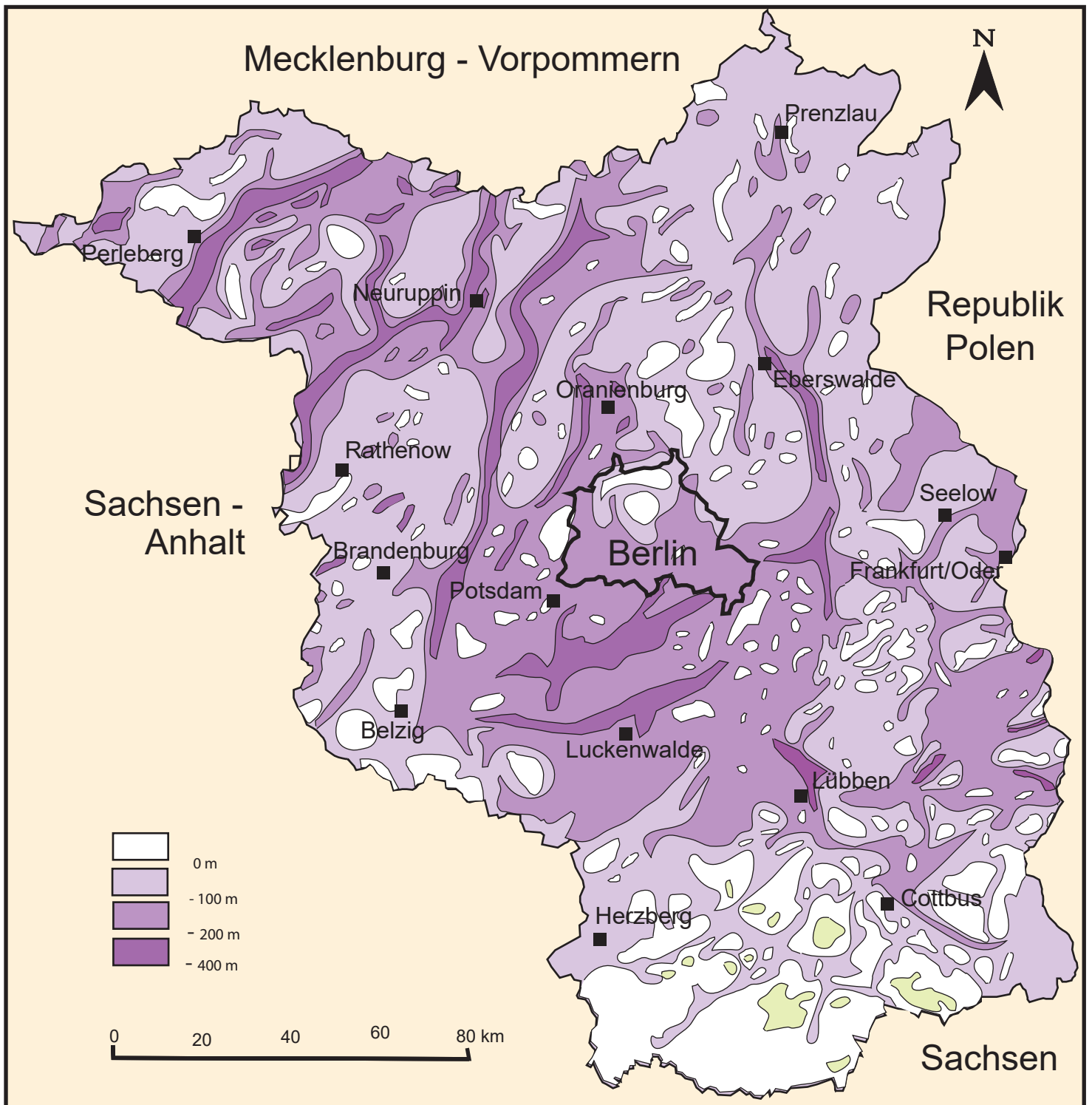
Abb. 25.34.1 Tiefenlage der Quartärbasisfläche im Bereich Brandneburgs nach G. BEST in H.-J. SCHLÜTER et al. 1997)
