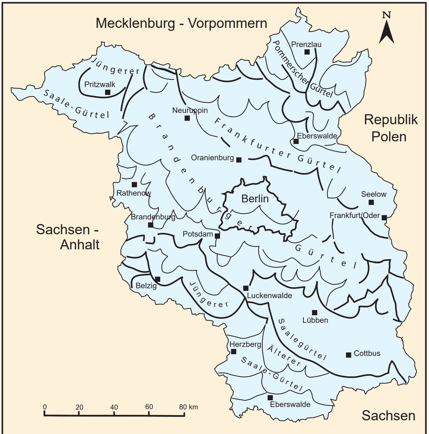
Abb. 25.34.2 Eisrandlagen in Brandenburg und ihre möglichen Verknüpfungen nach G. BEST in H.-J. SCHLÜTER et al. (1997)
