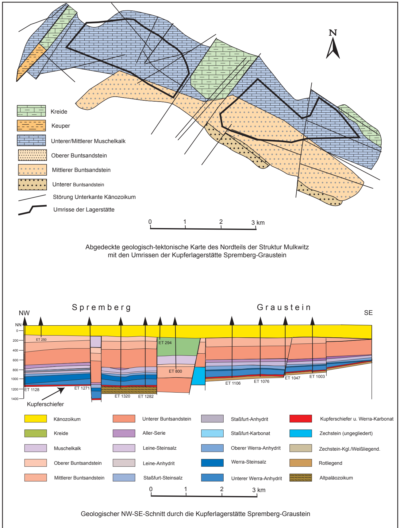
Abb. 25.35 Die Kupferlagerstätte Spremberg-Graustein (nach T. HÖDING 2014)
