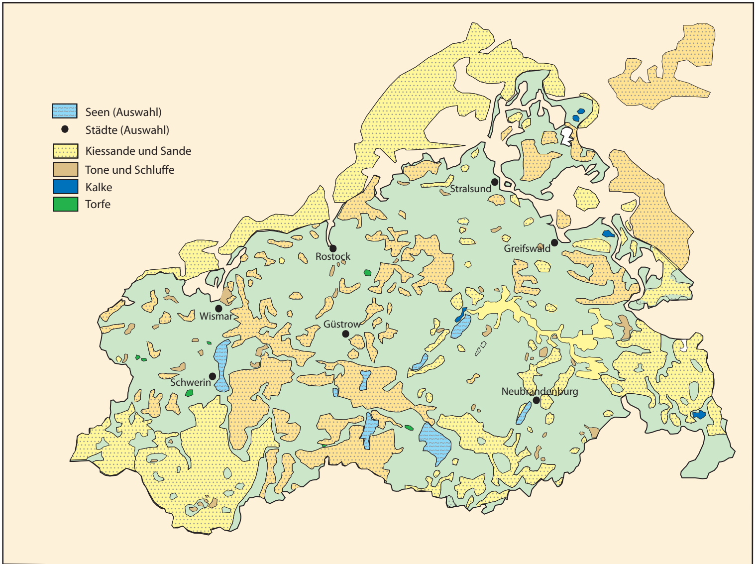
Abb. 25.36.7 Verbreitung oberflächennaher Rohstoffe in Mecklenburg-Vorpommern
