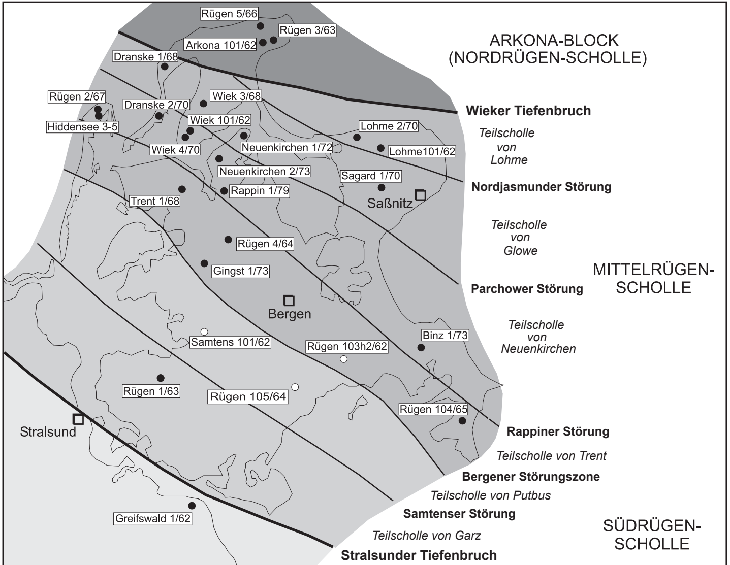
Abb.25.7 Bruchschollenbau des Präwestfalium im Inselbereich von Rügen-Hiddensee
