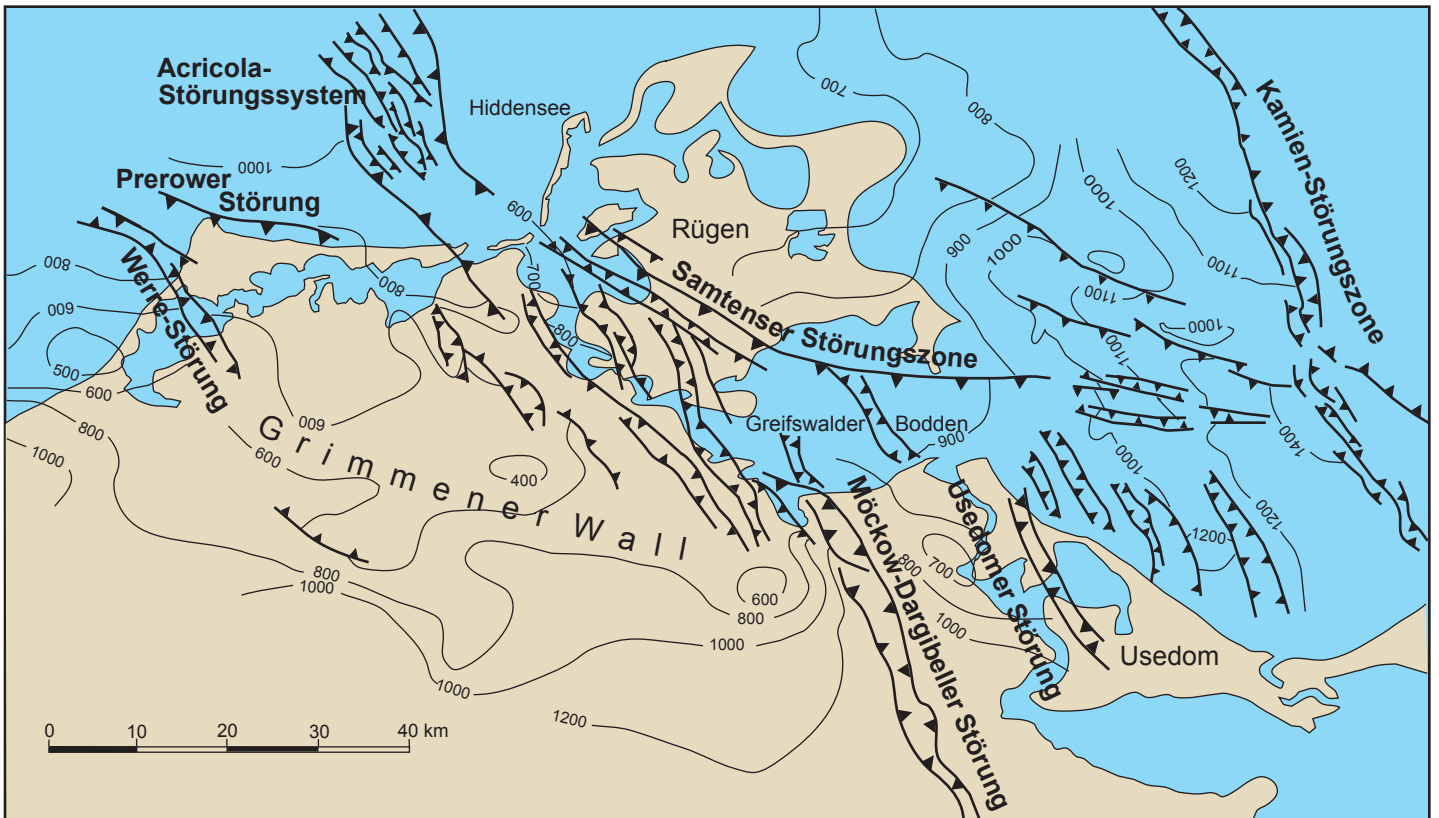
Abb. 25.8.2 Vorpommern-Störungssystem im Bereich der Insel Rügen und des angrenzenden Festlands (nach M. KRAUS & P. MAYER 2004)
