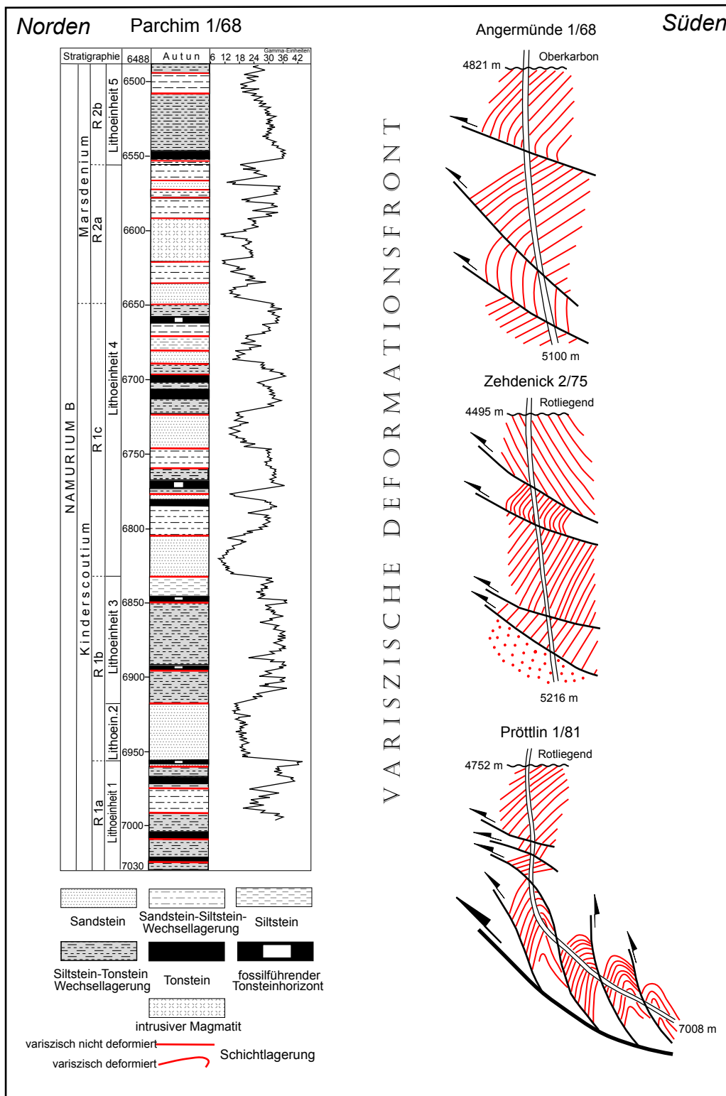
Abb. 25.9.1 Strukturelle Situation im Grenzbereich variszische Außenzone/prävariszisches Vorland (nach D. FRANKE et al. 2015b)
