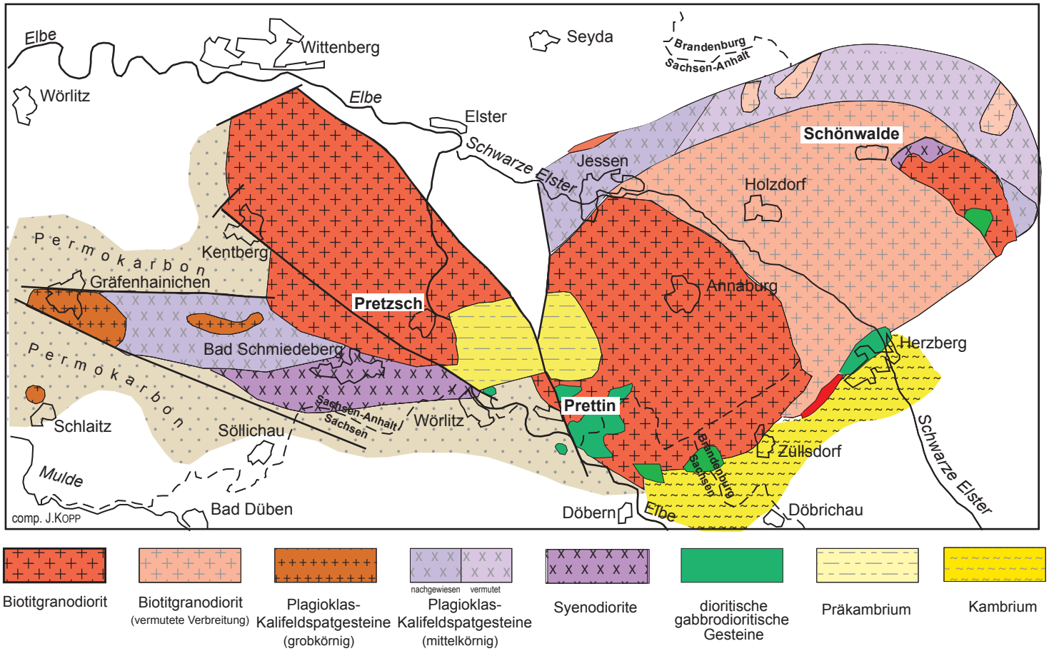
Abb. 25.9.2 Geologie des Plutonitmassivs von Pretzsch-Prettin-Schönwalde (nach J. KOPP 2008; D. FRANKE et al. 2015)
