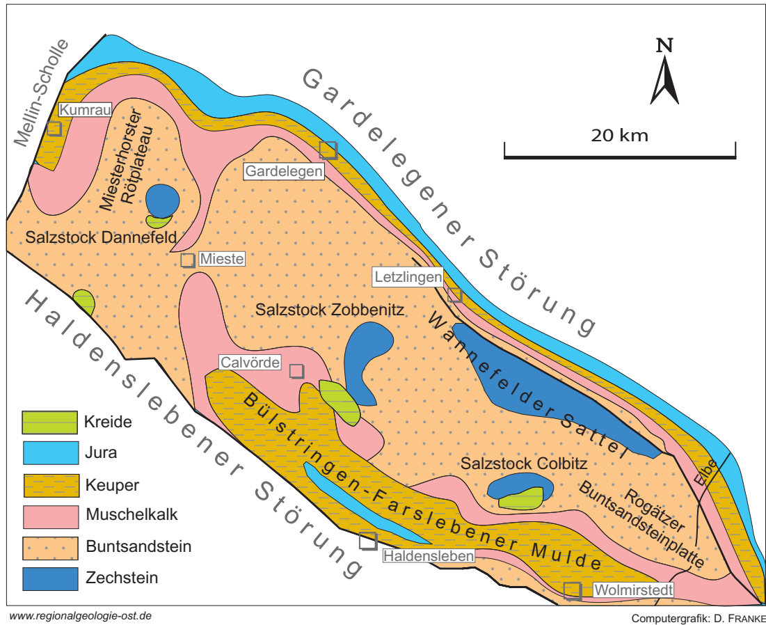
Abb. 26 Geologie des Präkänozoikum der Calvörder Scholle (nach G. SCHULZE 1964; G. MARTIKLOS et al. 2001)
