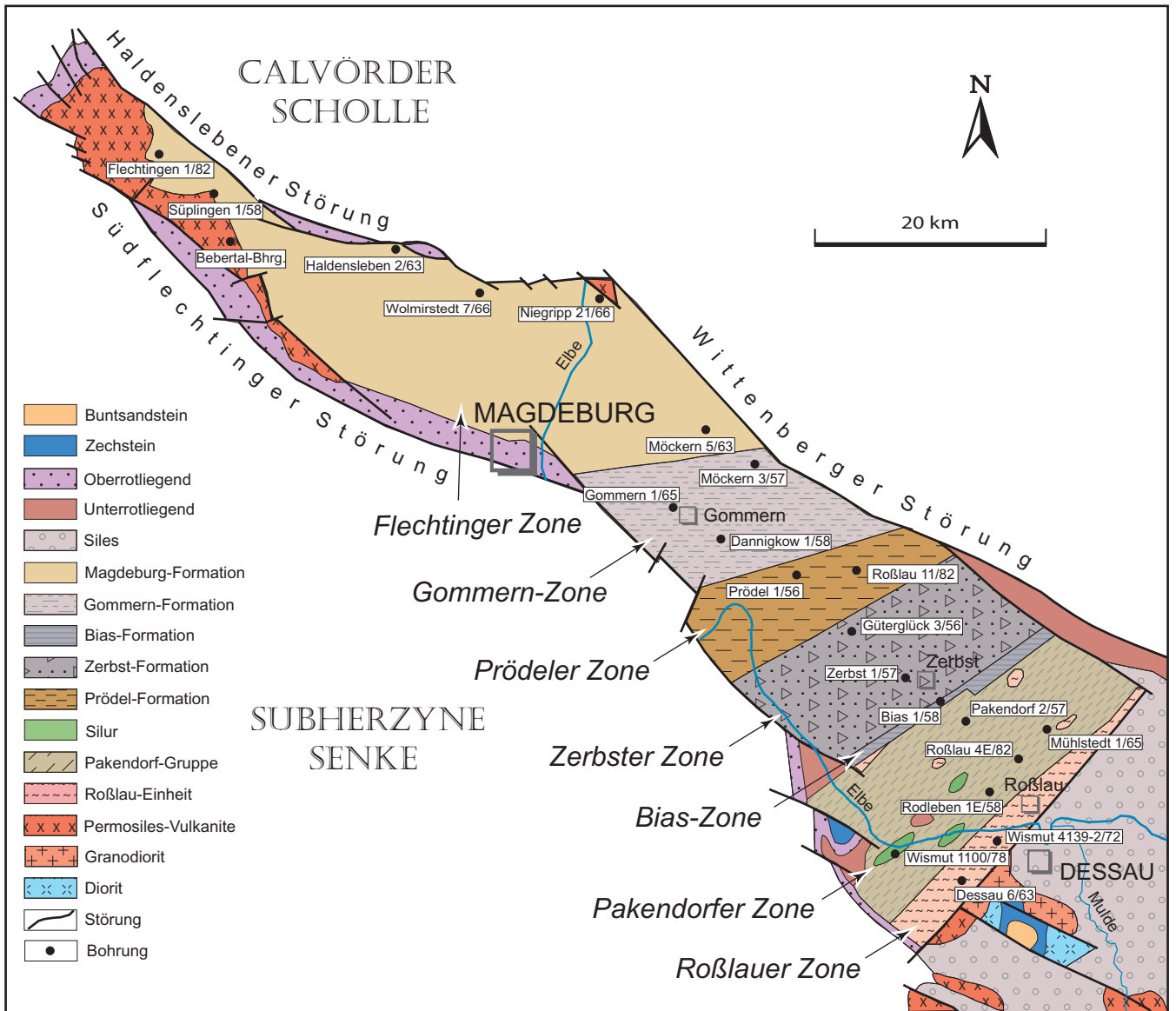
Abb. 27 Geologie des Präkämzoikum der Flechtingen-Roßlauer Scholle (nach G. MARTIKLOS et al. 2001; H.-J. PAECH et al. 2001, 2006)
