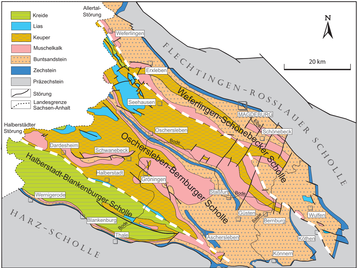
Abb. 28 Geologie der Subherzynen Senke Darstellung ohne känozoische Bildungen (nach G. MARTIKLOS et al. 2001)
