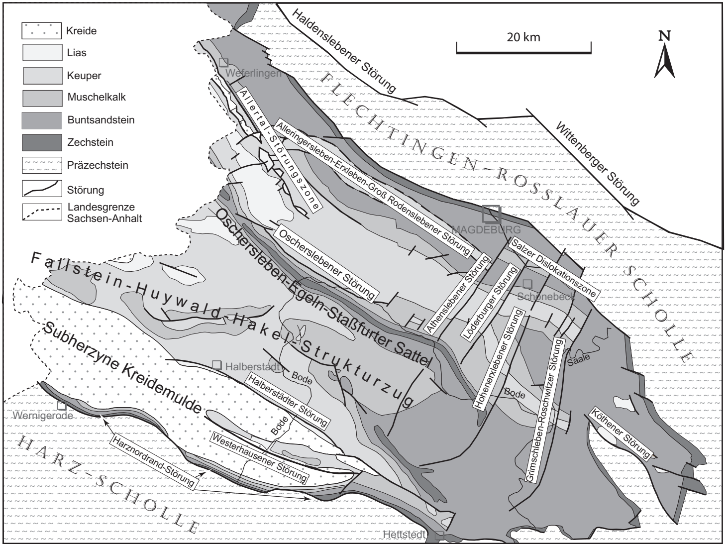
Abb. 28.2 Saxonisches Störungsmuster der Subherzynen Senke (nach G. MARTIKLOS et al. 2001; G. BEUTLER 2001) Zur Geologie der Subherzynen Senke vgl. Abb. 28, zum saxonischen Strukturbaue Abb. 28.1
