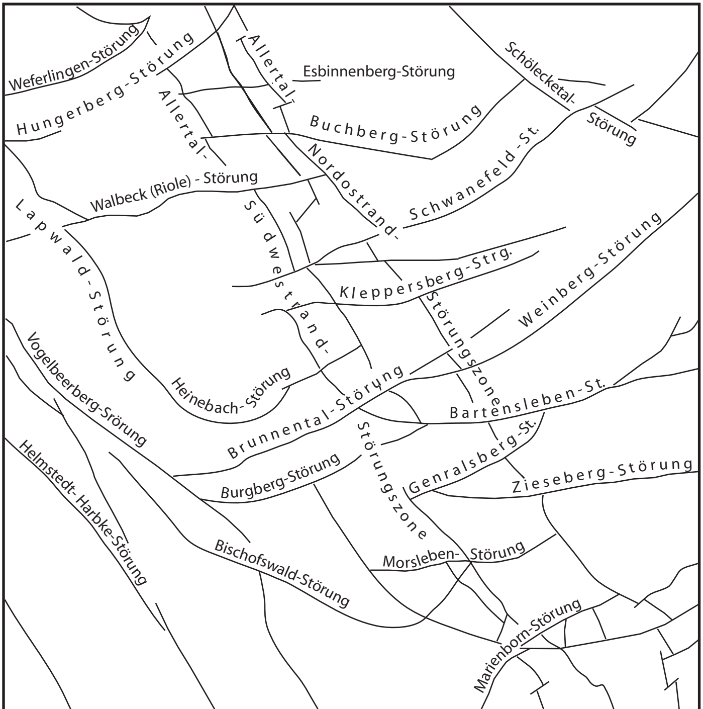
Abb. 28.2.2 Störungen im Suprasalinar der Allertal-Störungszone (nach C.-H. FRIEDEL, D. BALZER, L. STOTTMEISTER, G. BEUTLER & H.G.RÖHLING 2007)
