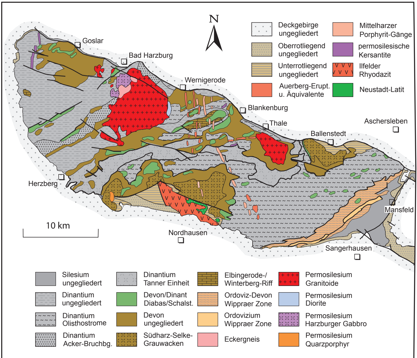
Abb. 29 Geologie des Harzes (nach C. HINZE et al. 1998; G. MARTIKLOS et al. 2001)
