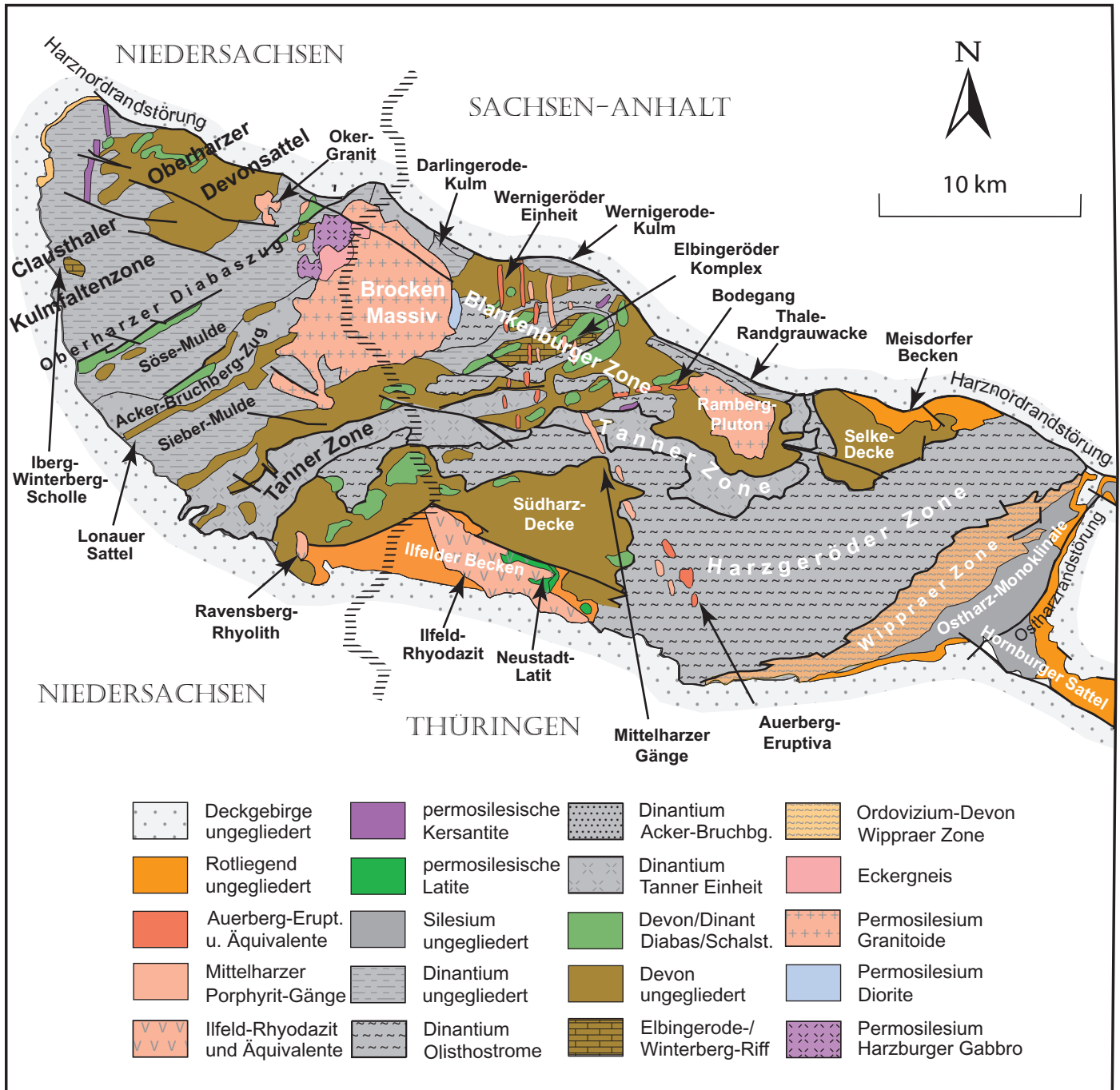
Abb. 29.1 Regionaleinheiten des Harzes (im Wörterbuch sind nur Einheiten des Ostharzes enthalten) (nach K. MOHR 1993; C. HINZE et al. 1998; G. MARTIKLOS et al. 2001; M. SCHWAB 2008a)
