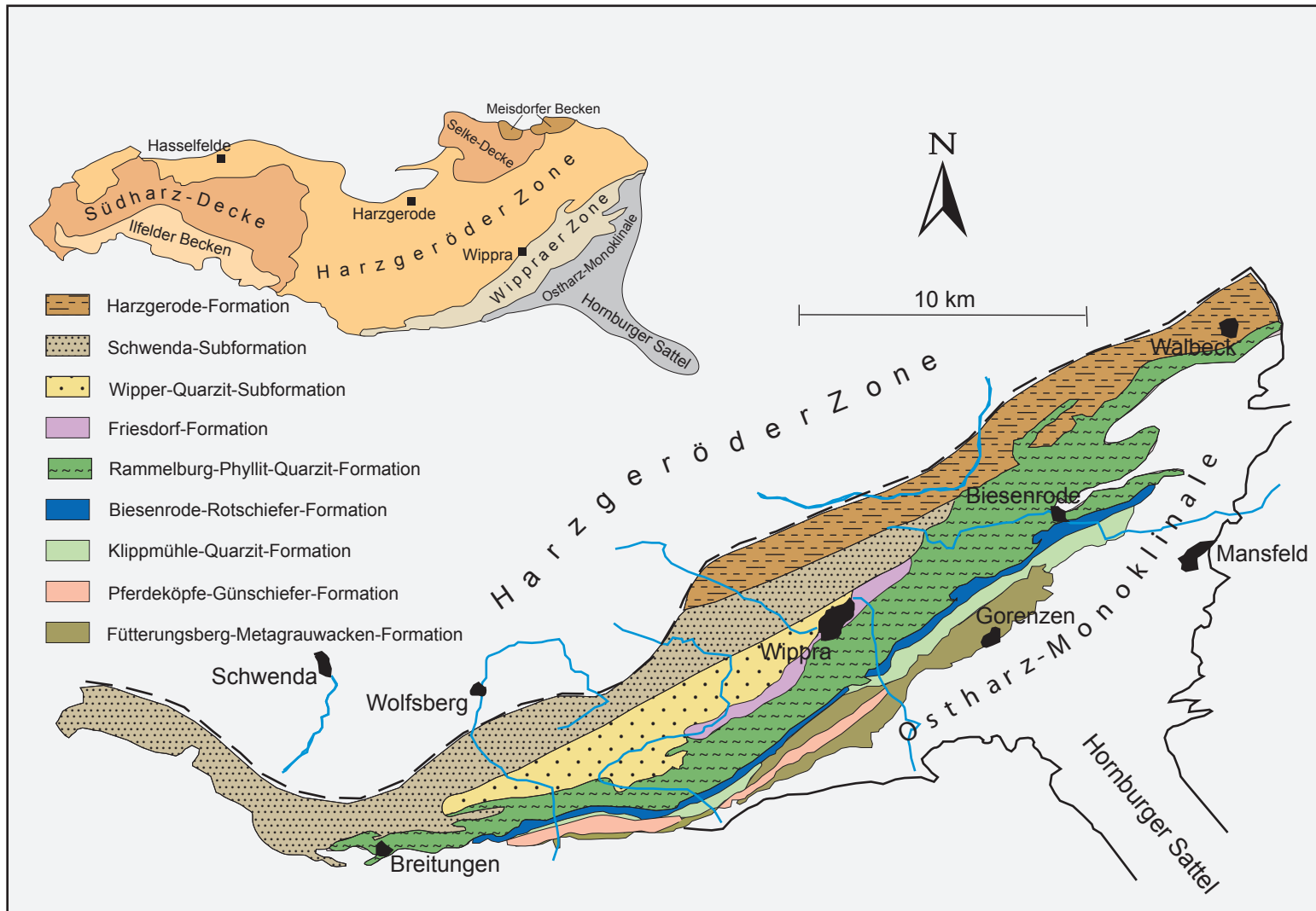
Abb. 29.11 Geologie der "Metamorphen Zone" des Harzes (nach TH. MÜLLER, H. HEINICH & D. MERTMANN 2012)
