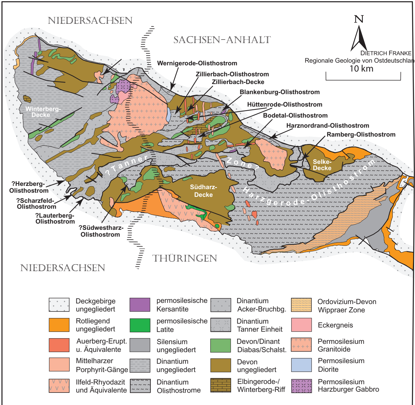
Abb. 29.2 Allochthone und olistostromale Bildungen des Harzes (im Wörterbuch sind nur Begriffe des Osthazes enthalten) (nach H. LUTZENS & M. SCHWAB 1972; C. HINZE et al. 1998; G. MARTIKLOS et al. 2001; M. SCHWAB 2008a)
