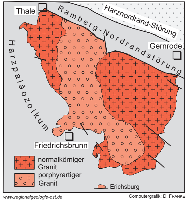
Abb. 29.6 Geologie des Ramberg-Plutons (nach R. BENEK 1967, C. HINZE et al. 1998)
