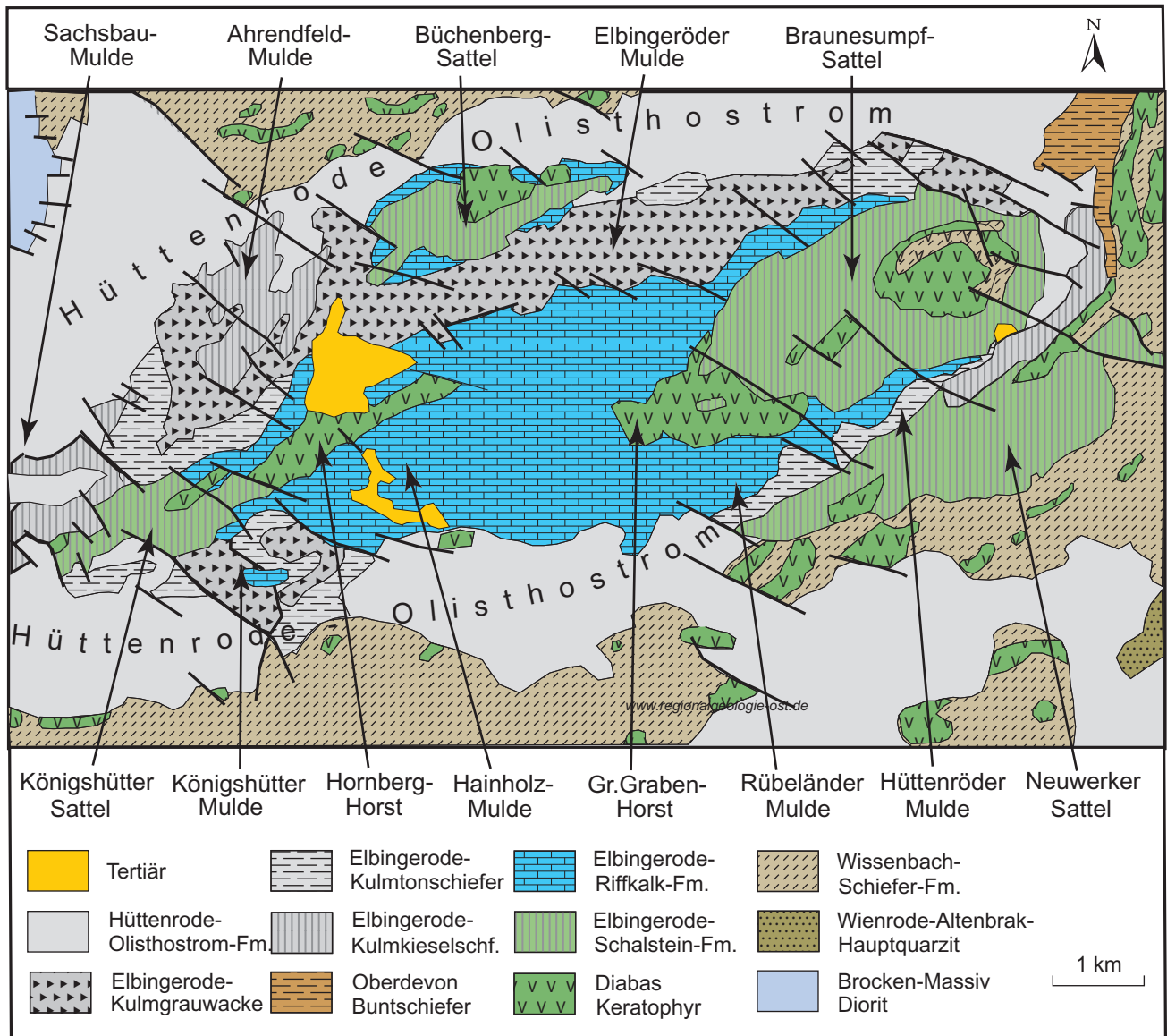
Abb. 29.7 Geologie des Elbingeröder Komplexes Darstellung ohne Mittelharzer Eruptivgesteinsgänge (nach H. LUTZENS 1979; K. RUCHHOLZ & H. WELLER 1988, 1991a; C. HINZE et al. 1998)
