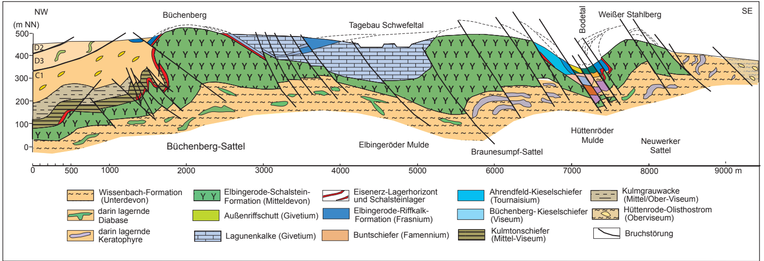
Abb. 29.9 Geologischer Profilschnitt durch den Elbingeröder Komplex
