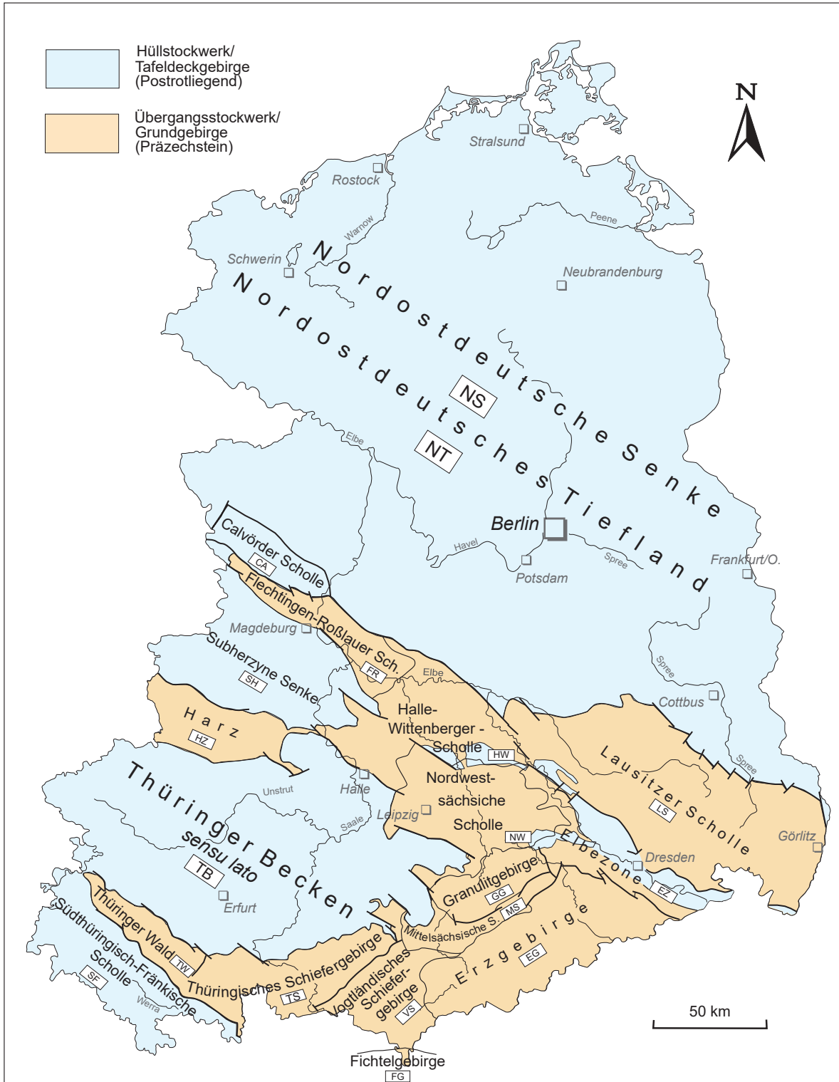
Abb. 3 Regionalgeologische Grundgliederung Ostdeutschlands (im Wesentlichen nach Geologie-Standard TGL 34331/01 1983; publiziert in G. KATZUNG & G. EHMKE 1993, D. FRANKE (2007) Die Kürzel kennzeichnen im Wörterbuch die Zuordnung der einzelnen Begriffe zu den entsprechenden Regionaleinheiten
