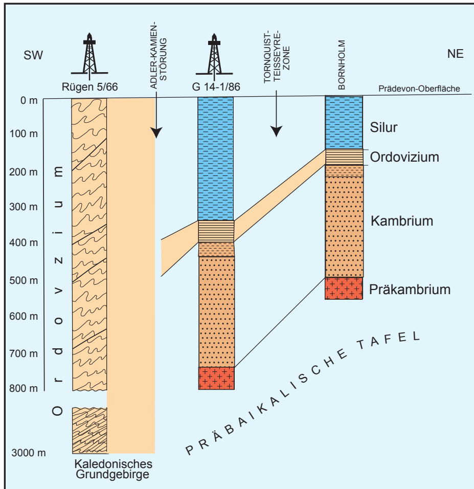
Abb. 3.1.1 Übergangsbereich Rügen-Kaledoniden/präbaikalische Tafel
