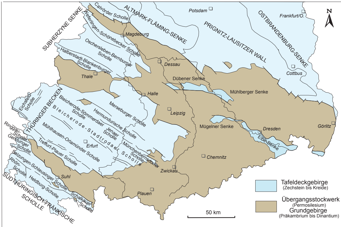
Abb. 3.2 Senken und Schollen des Tafeldeckgebirge im Südtteil Ostdeutschlands (nach Geologie-Standard TGL 34331/01 1983; publiziert in G. KATZUNG & G. EHMKE/Hrsg. 1993; G. SEIDEL 2003, 2004)
