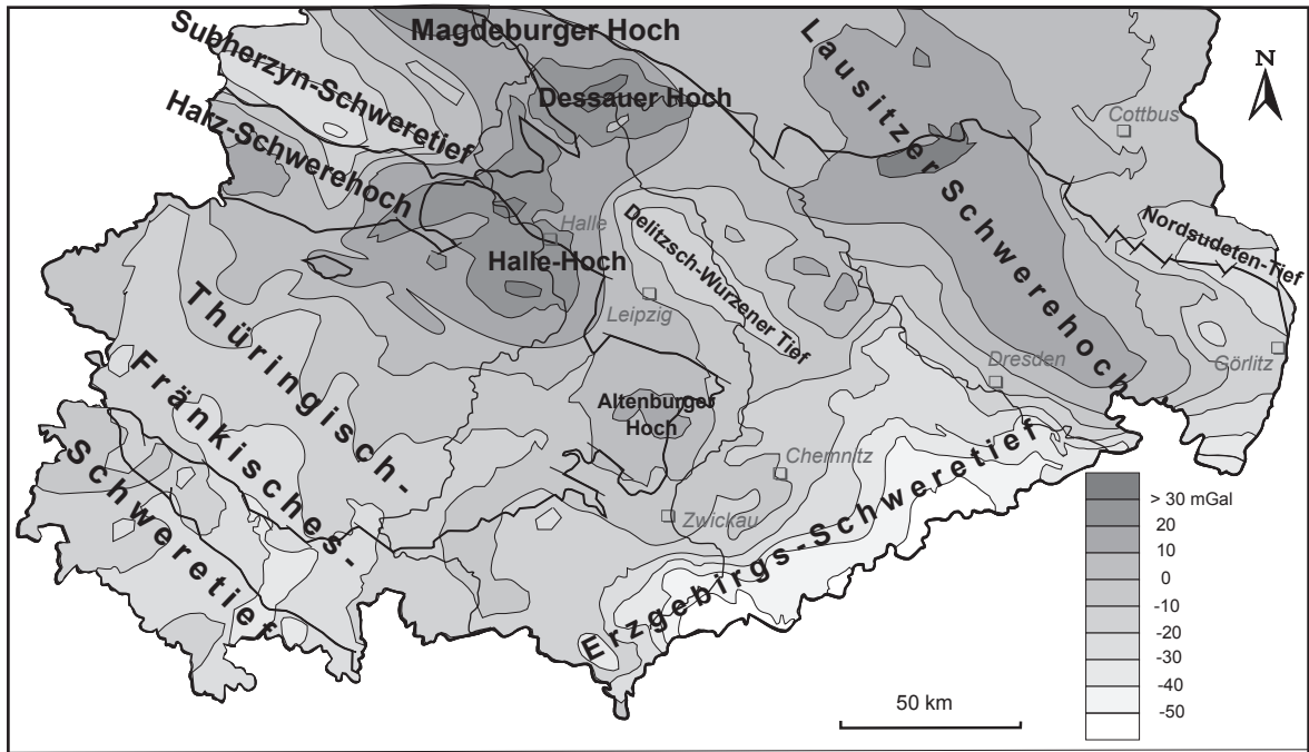
Abb. 3.3 Isanomalien der Bouguerschwere im Bereich des Sächsisch-Thüringischen Schollenkomplexes - Übersichtsdarstellung
