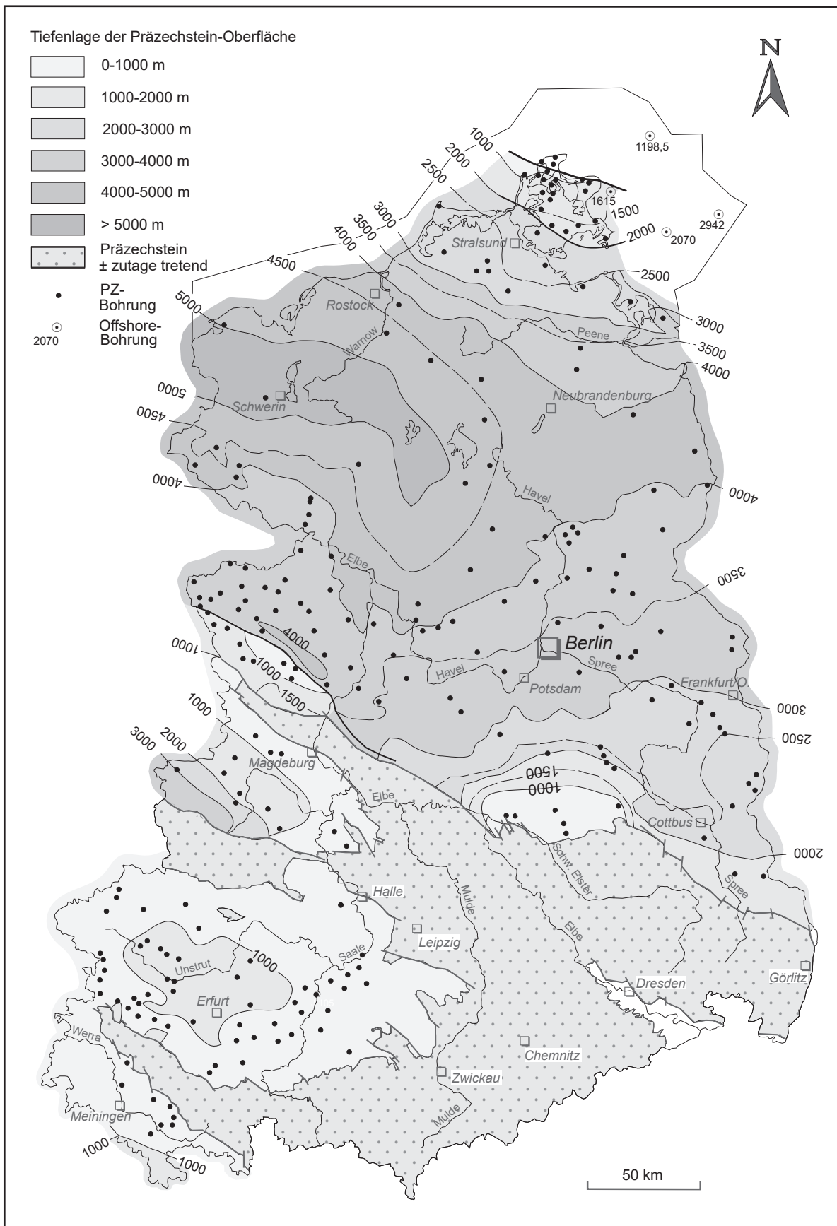
Abb. 3.3 Tiefenlage der Präzechstein-Oberfläche in den vom Tafeldeckgebirge überlagerten Senkenbereichen Ostdeutschlands (nach Ergebnissen der Reflexionsseismik und ausgewählter Tiefbohrungen) (aus D. FRANKE (2007))
