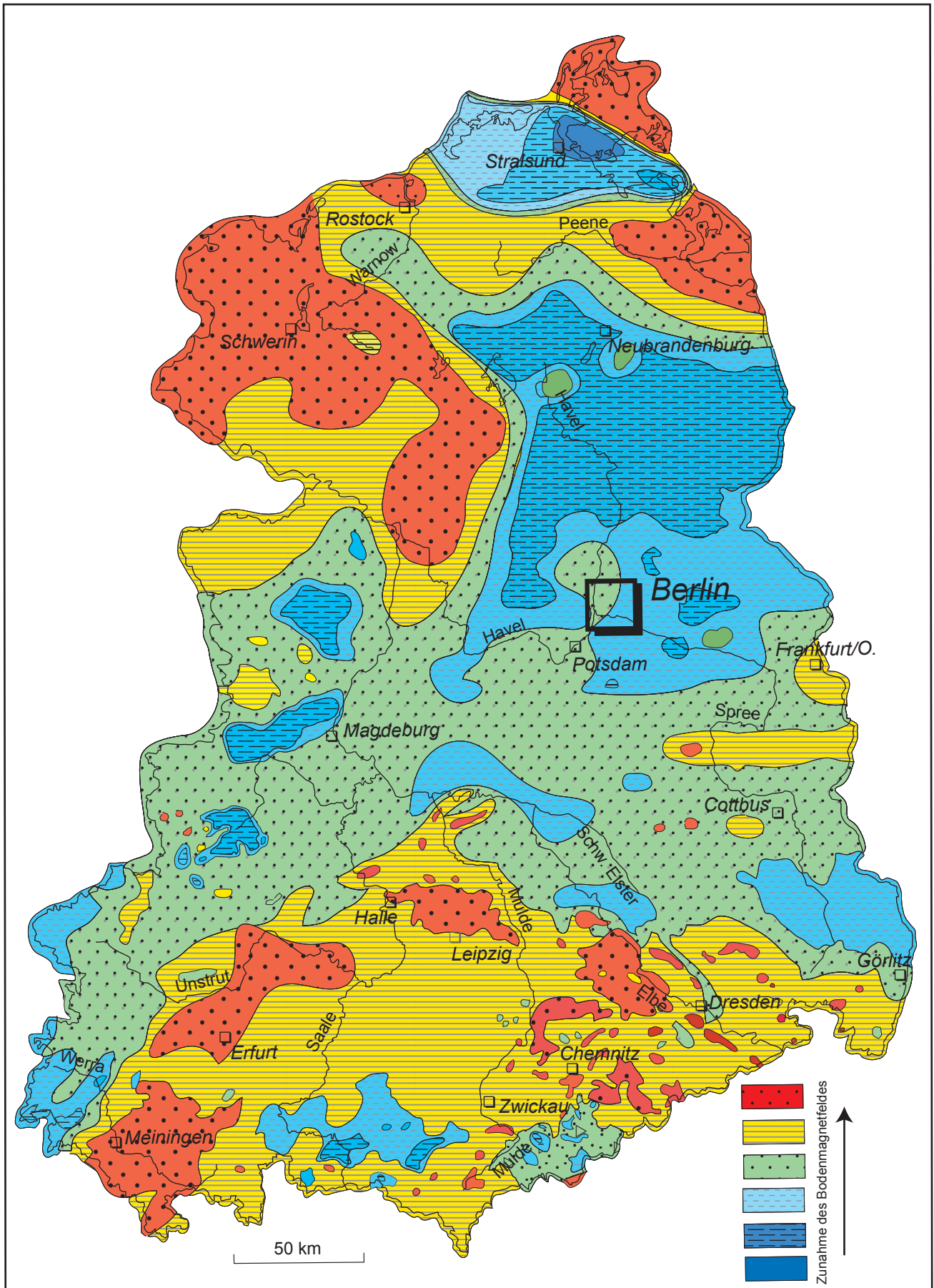
Abb. 3.4 Übersichtskarte des Magnetfeldes im Bereich Ostdeutschlands (nach Leibnitz-Institut für Angewandte Geophysik )
