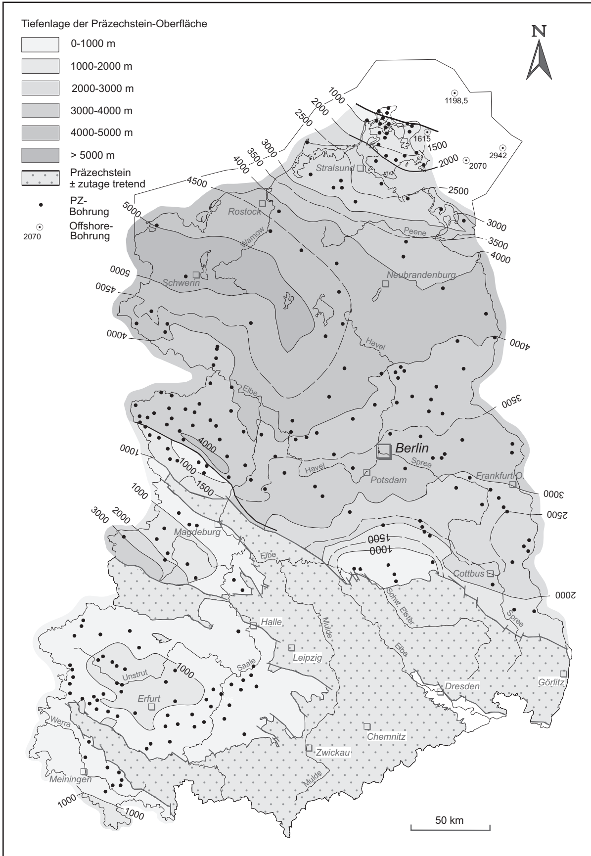
Abb. 3.7 Tiefenlage der Präzechestein-Oberfläche in den vom Tafeldeckgebirge überlagerten Senkenbereichen Ostdeutschlands (nach Ergebnissen der Reflexionsseismik und ausgewählter Tiefbohrungen)
