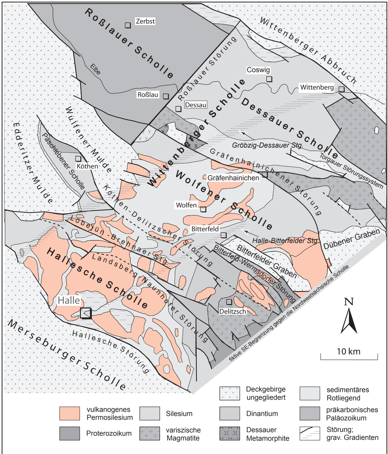
Abb. 30.1 Strukturbaue der Halle-Wittenberger Scholle Darstellung ohne känozoische Bildungen (nach G. MARTIKLOS et al. 2001; G. BEUTLER 2001; I. RAPPSILBER 2003)
